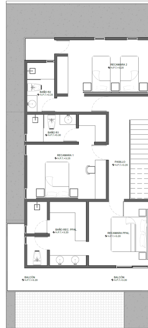
PLANTA ALTA
