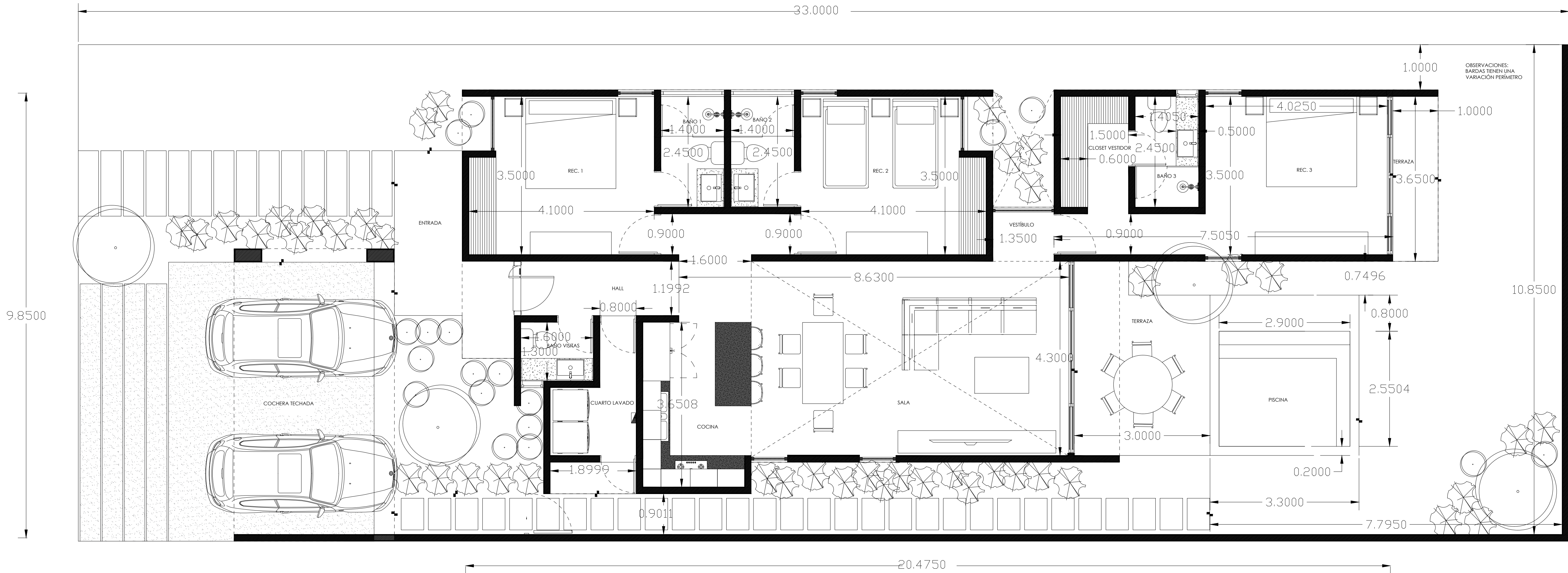
1 | ARQ_PLANTA BAJA ESC: 1:50
