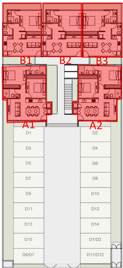
PLANTA BAJA
