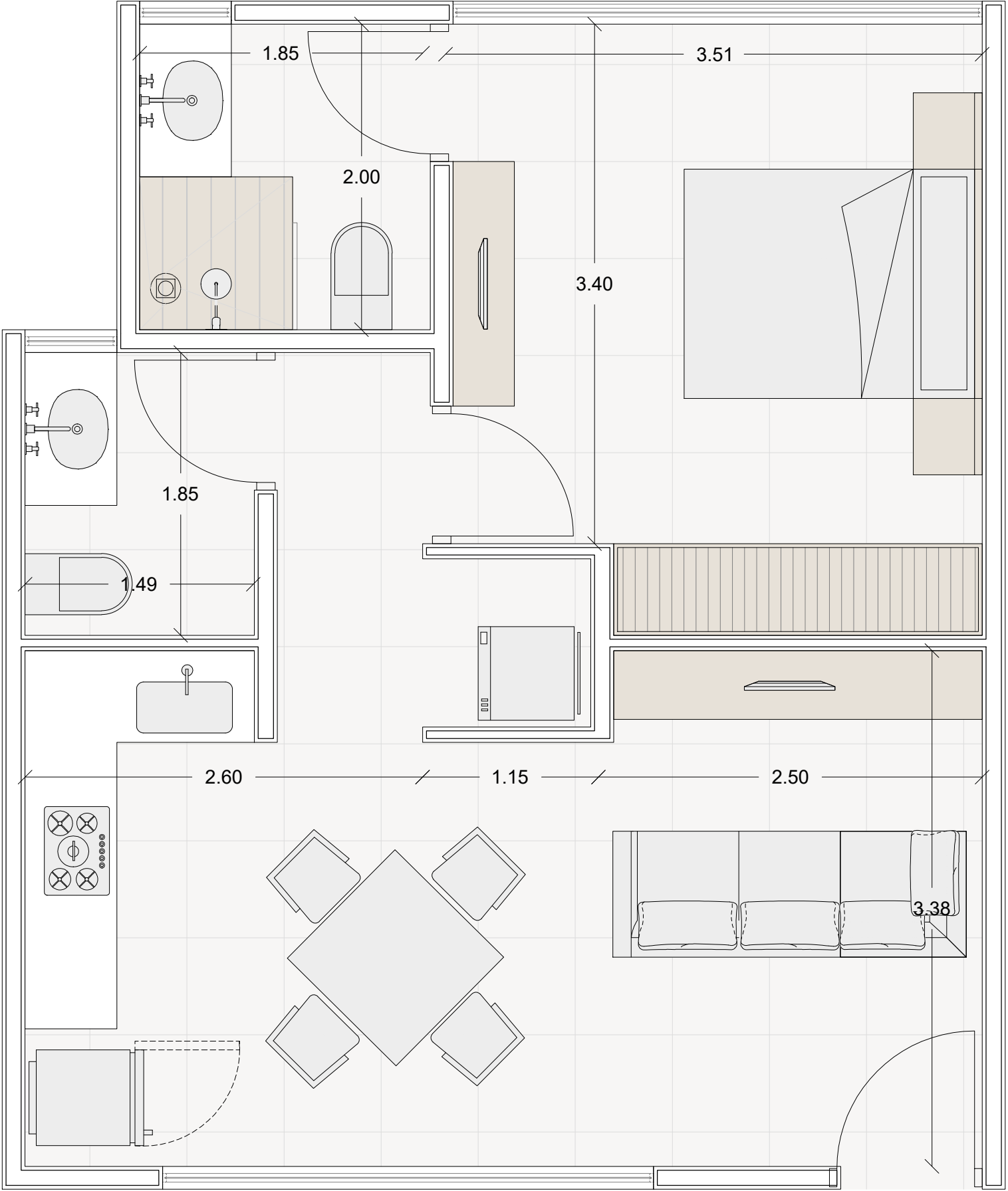
DEPARTAMENTO TIPO B
