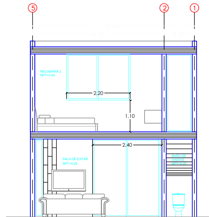
CORTE C - C'
