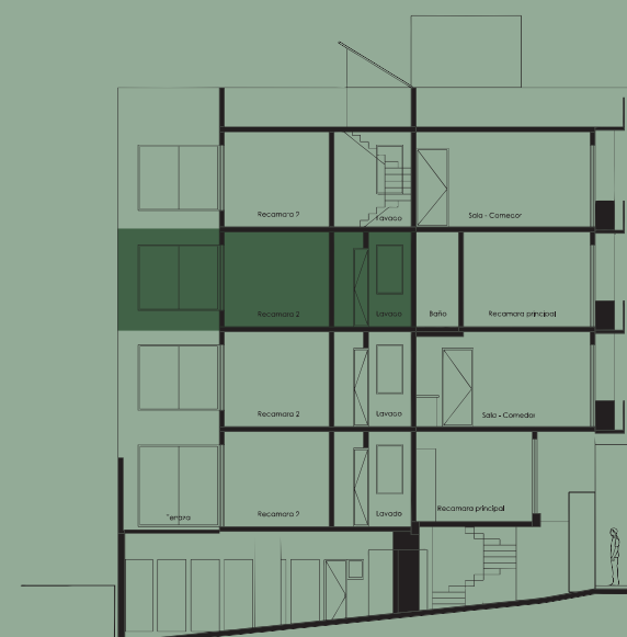
nivel + 3
