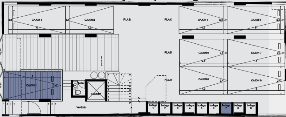
Planta sótano - Cajón 1 y Bodega 7
