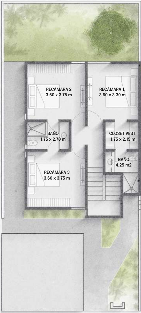
PLANTA ALTA
