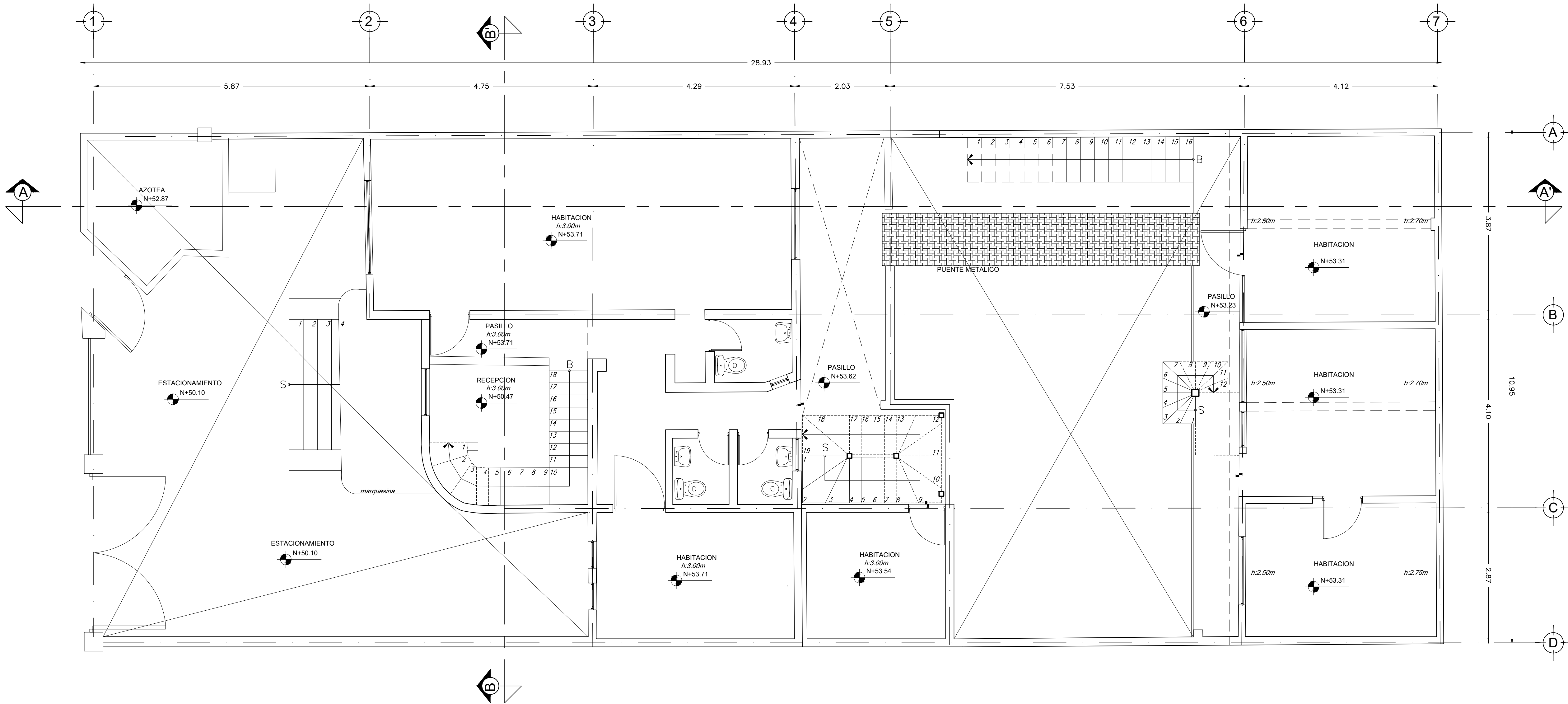
PLANTA 1ER NIVEL
