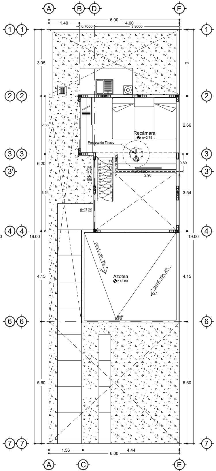
Planta Arquitectonica Alta
