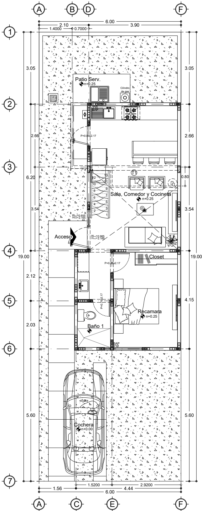
Planta Arquitectonica Baja
