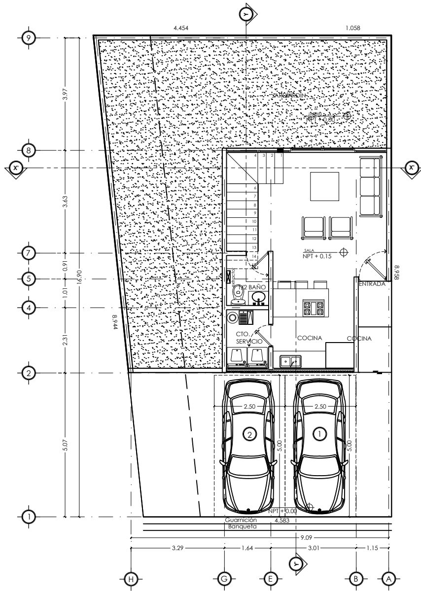
PROYECTO ARQUITECTÓNICO ESC 1:75 PLANTA BAJA (P1)
