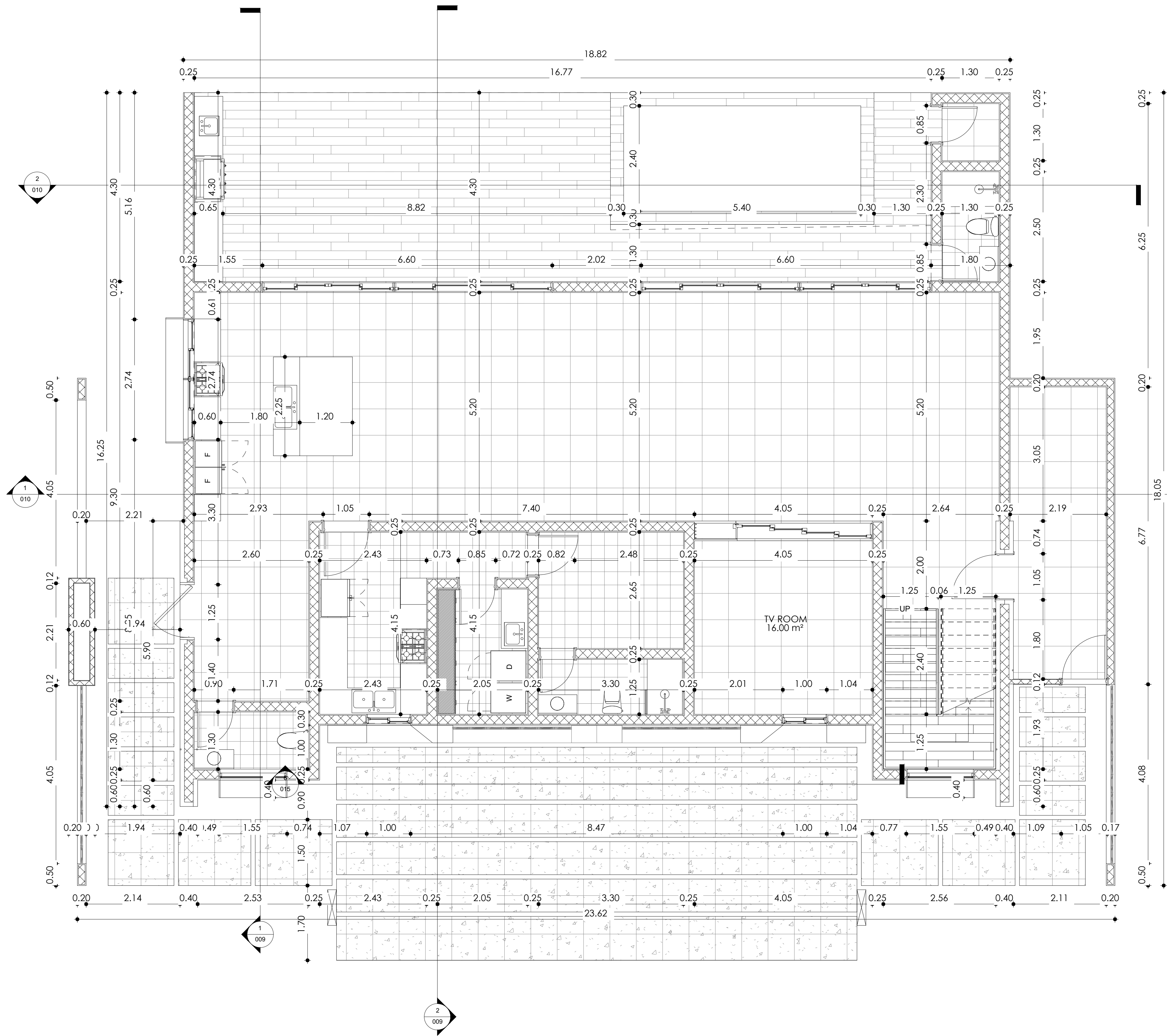
PLANTA DIMENSIONADA N01 - VILLAS
