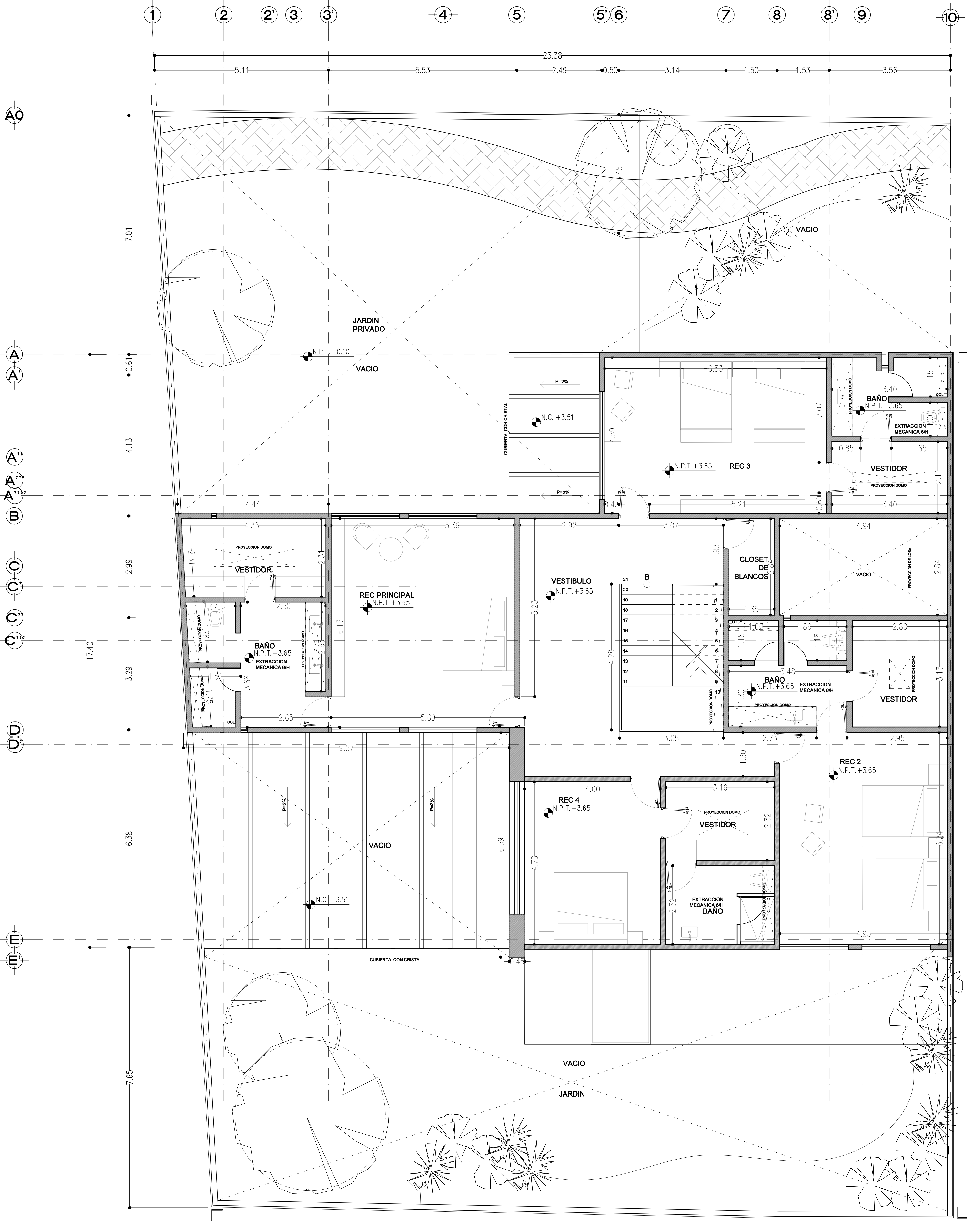
PLANTA ALTA MODIFICADA 4a RECAMARA
