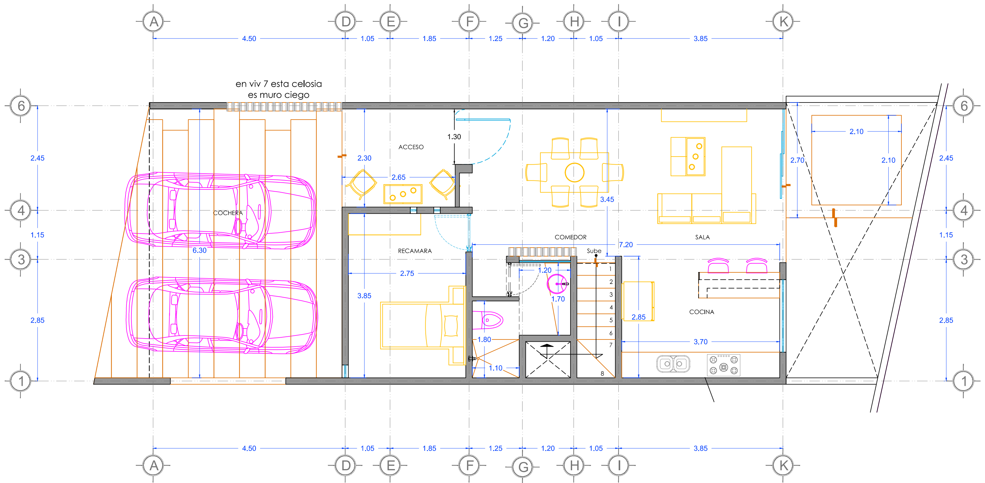
PLANTA BAJA
