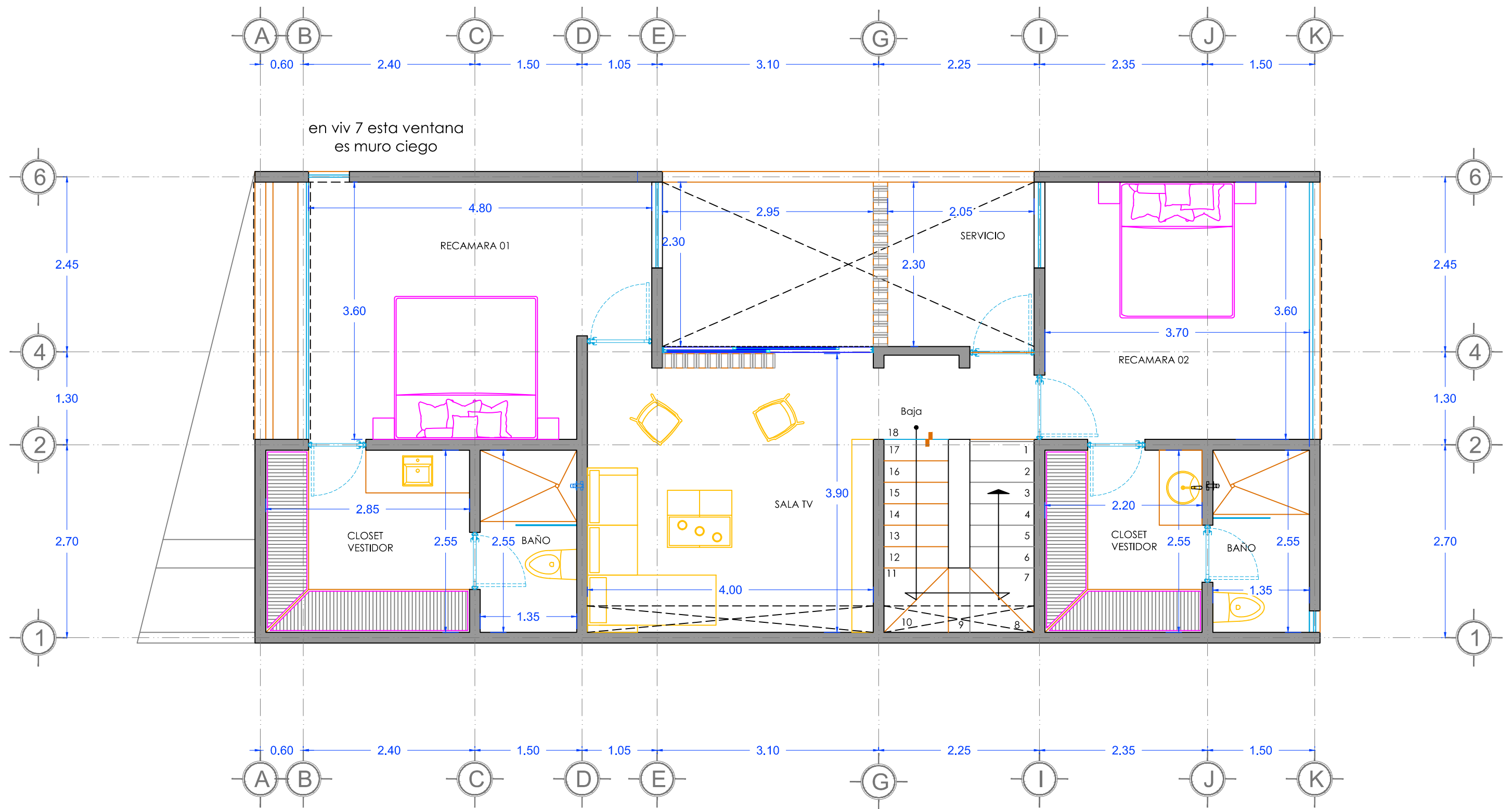
PLANTA ALTA
