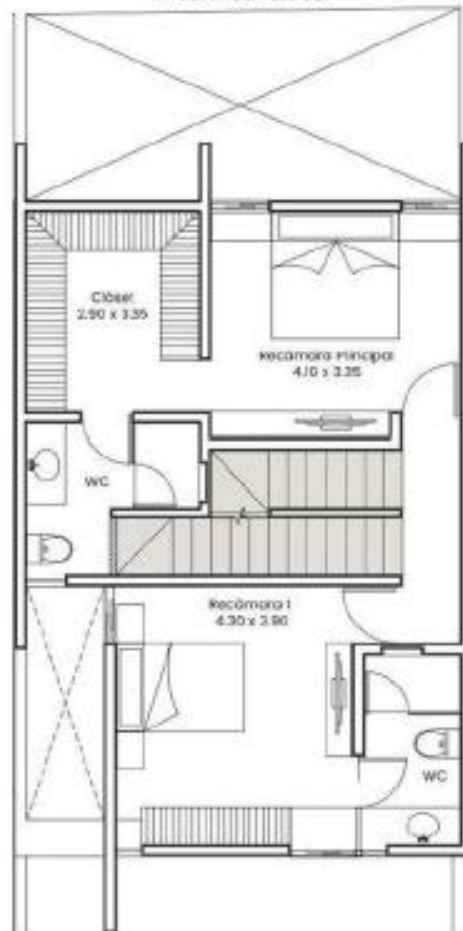
Planta alta
