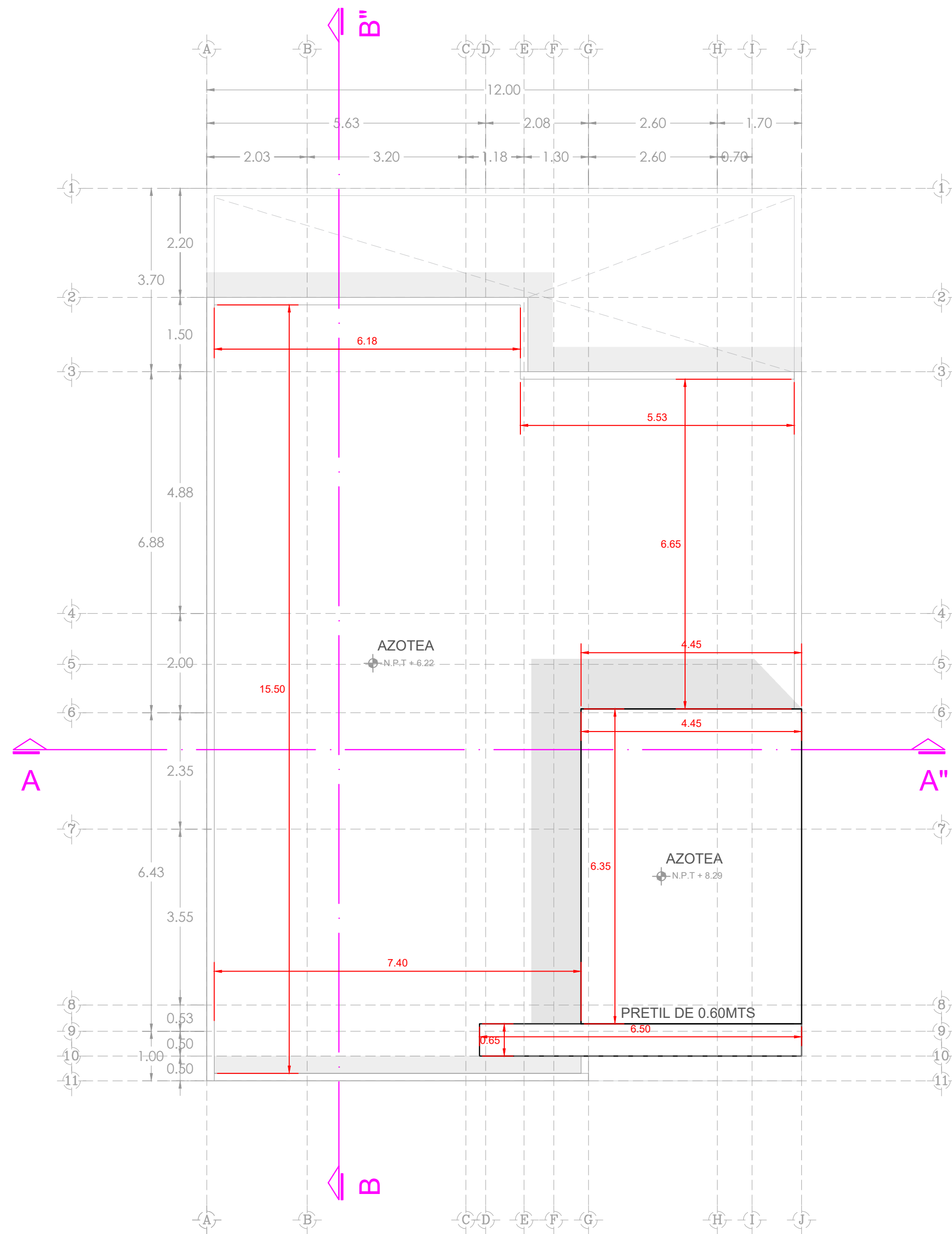
NIVEL DE AZOTEA CASA DELUXE ANA 177.97M2
