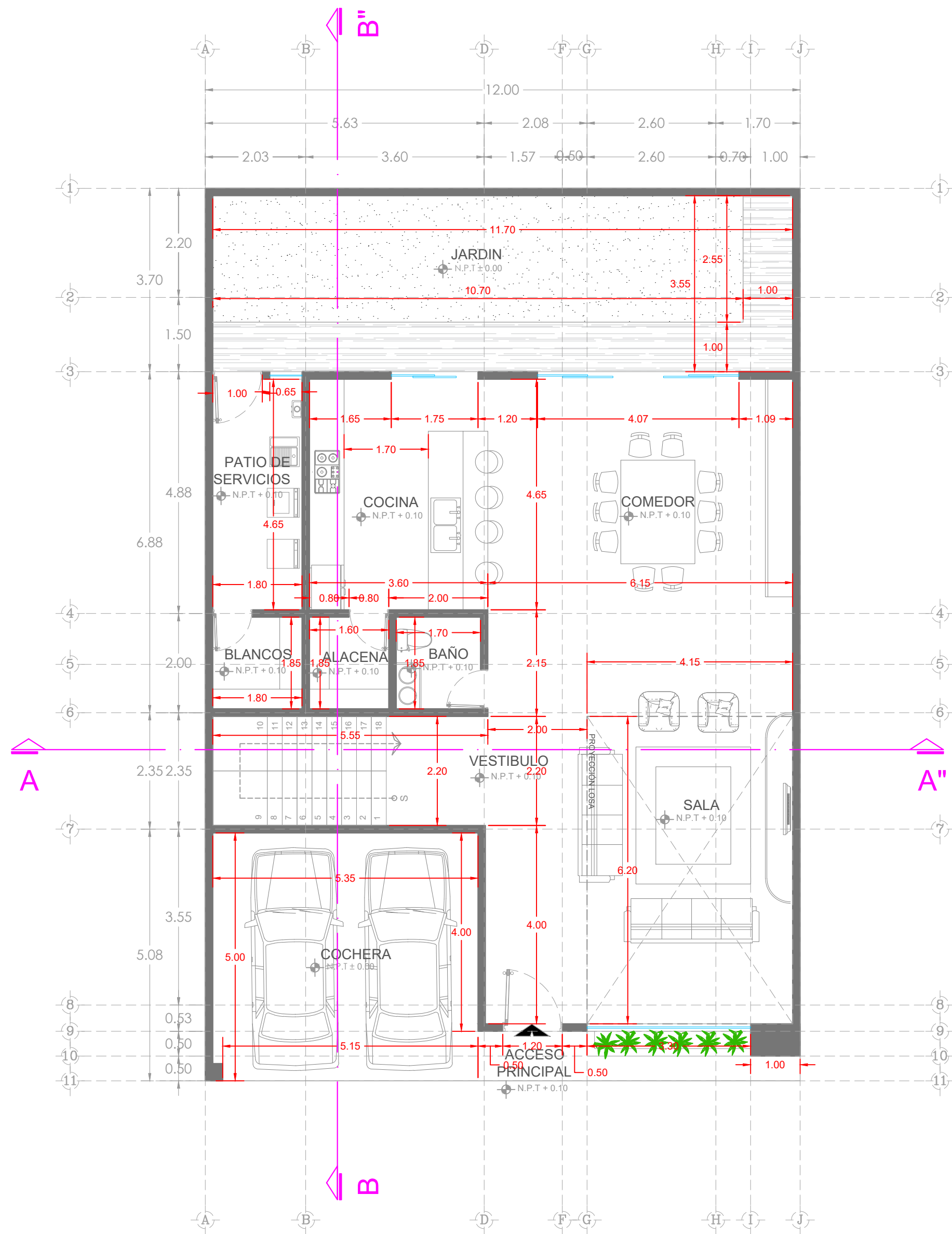
NIVEL DE PLANTA BAJA CASA DELUXE ANA 216M2
