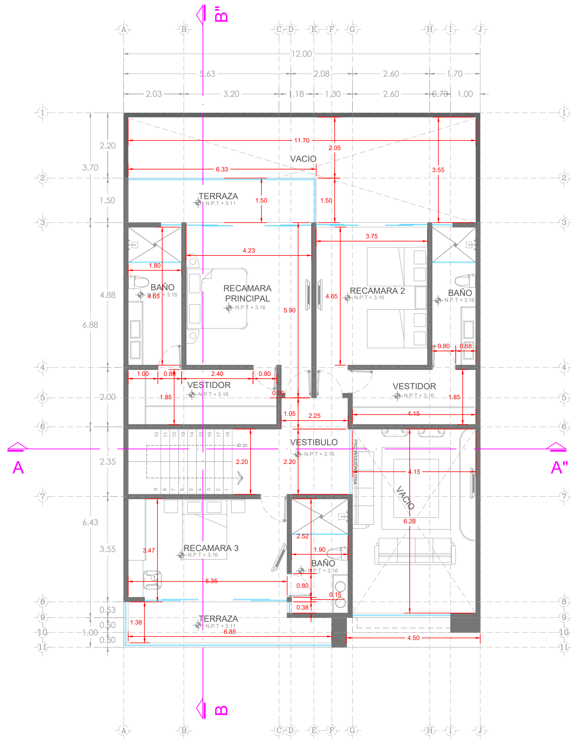
NIVEL 01 CASA DELUXE ANA 177.31M2
