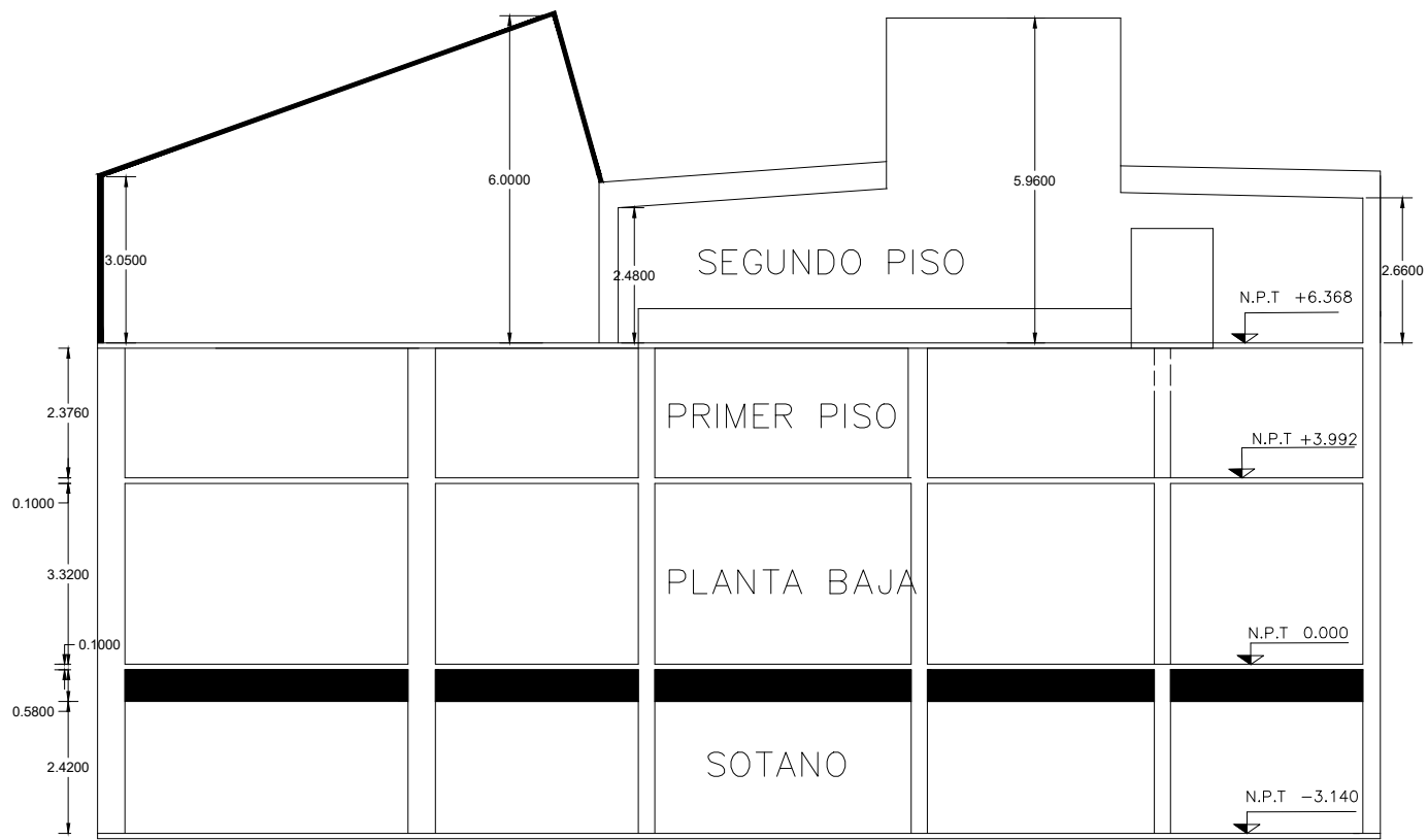
CORTE ESQUEMATICO
