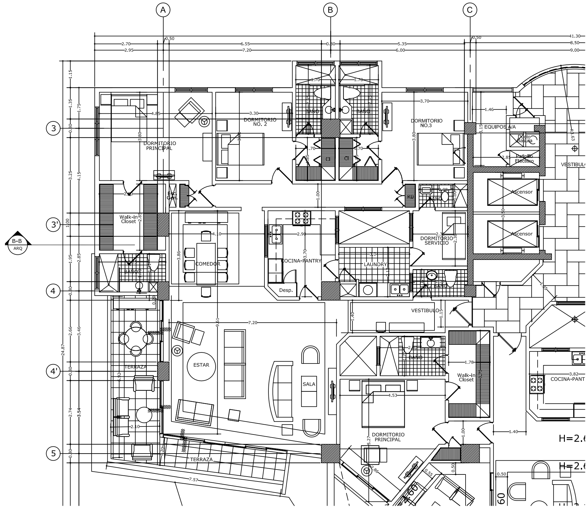
1 PLANTA ARQUITECTONICA - Apt. Oeste A-07 Escala 1:100
