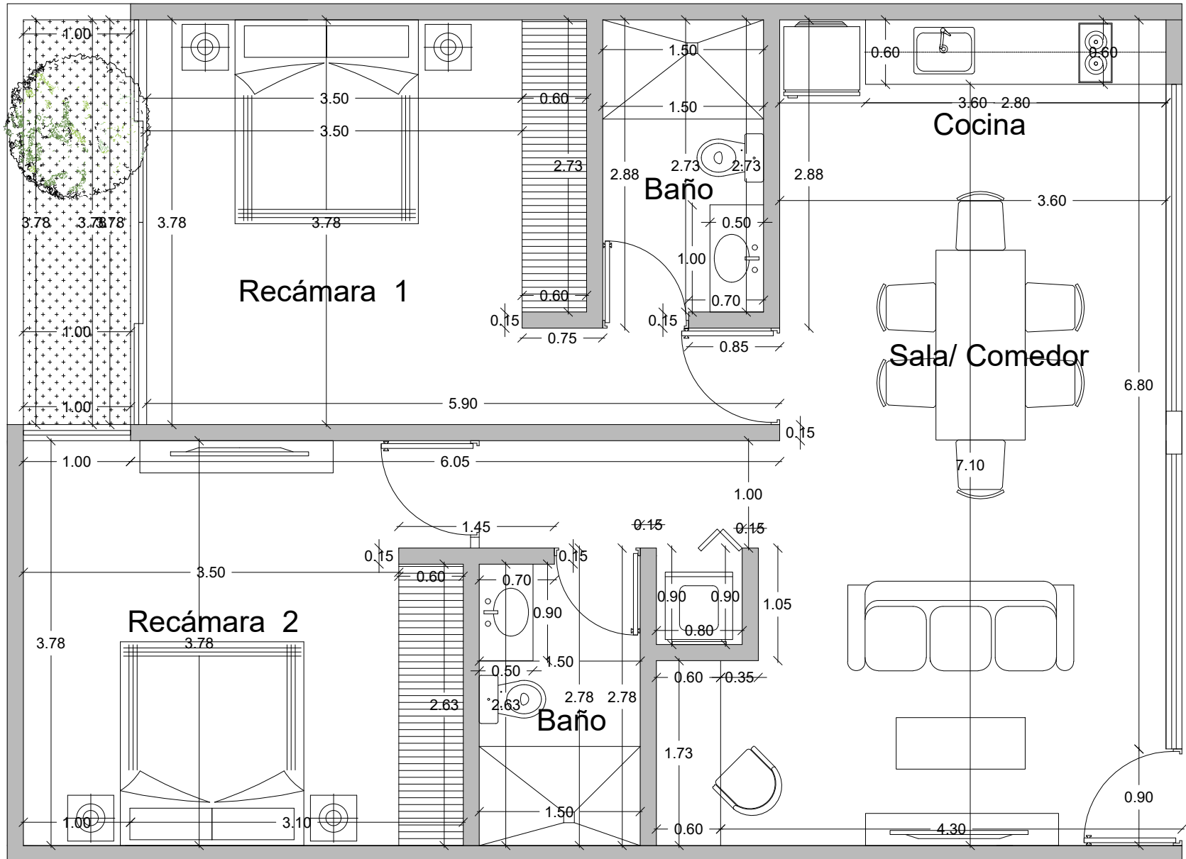
DEPARTAMENTO TIPO B 80.00 mts 2
