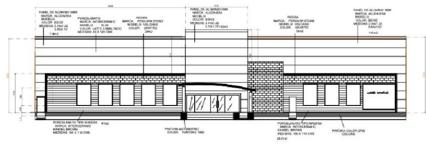
Elevación Principal
