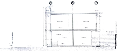
SECCIÓN LONGITUDINAL
