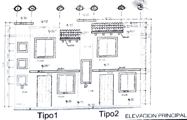
ELEVACIÓN PRINCIPAL
