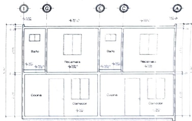
SECCIÓN TRANSVERSAL
