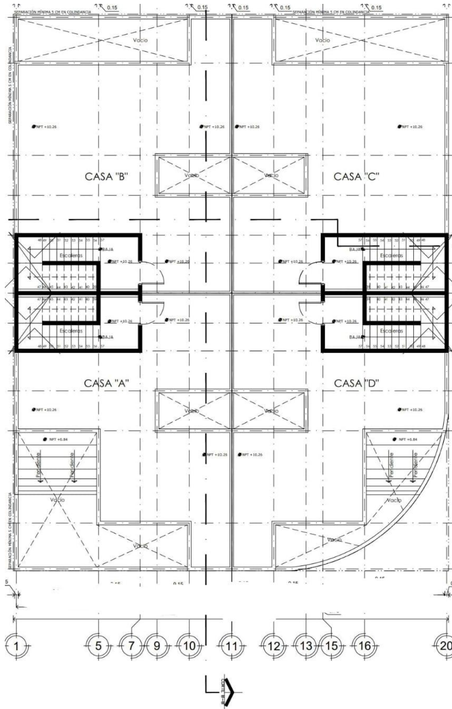
Planta Arquitectónica Azotea
