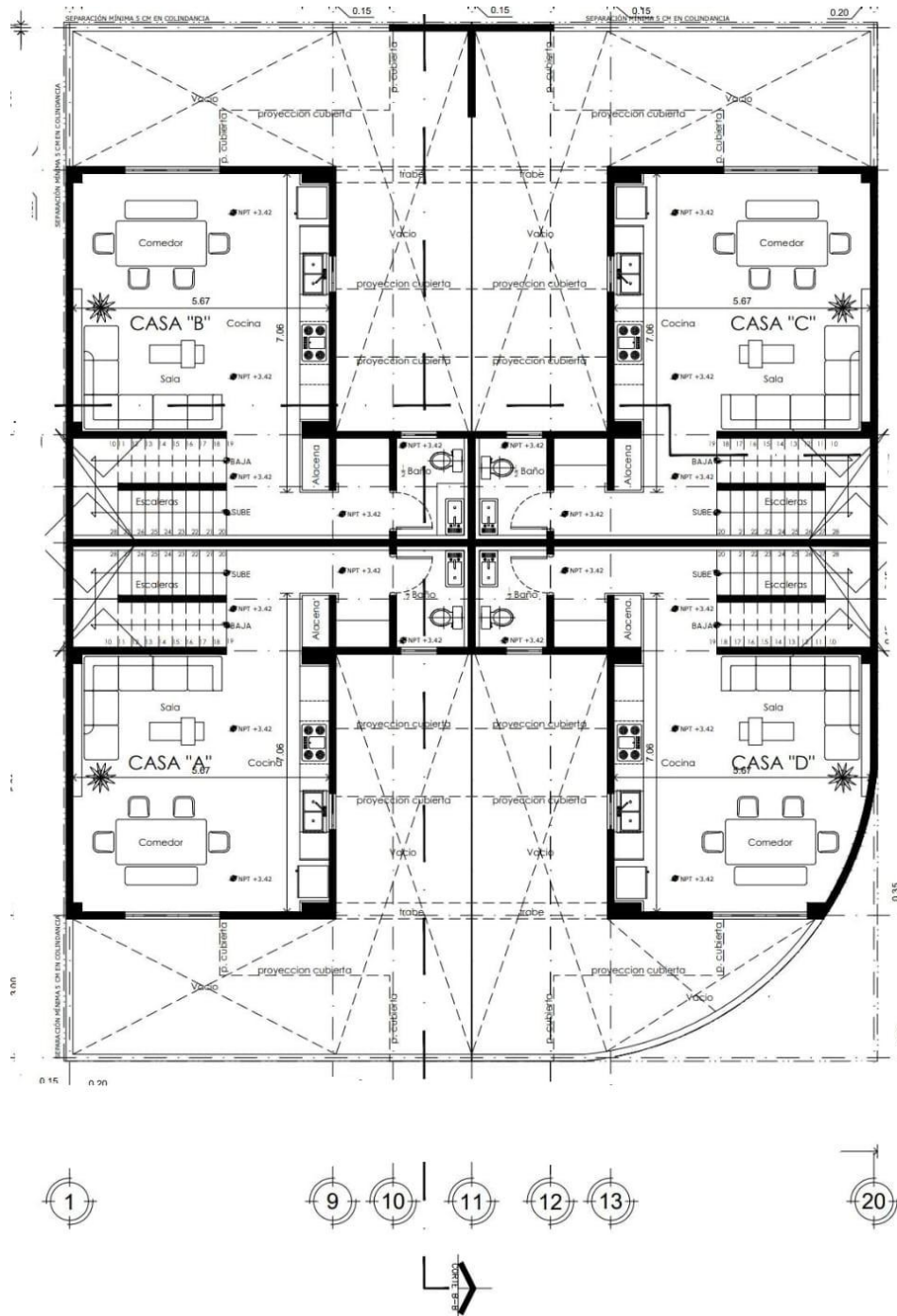
Planta Arquitectónica Baja
