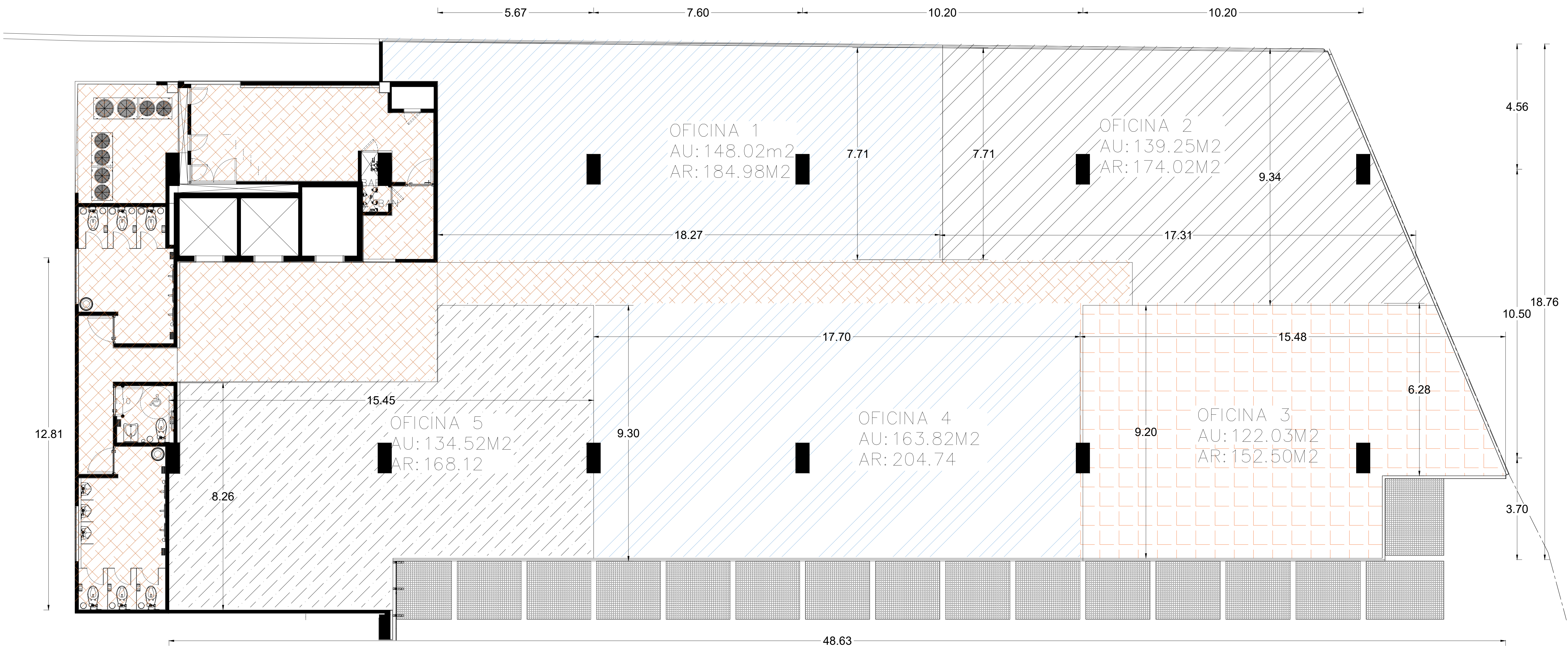
PLANTA TIPO OFICINAS NIVEL 2, 3, 4, 5, 6, 7 Y 8
