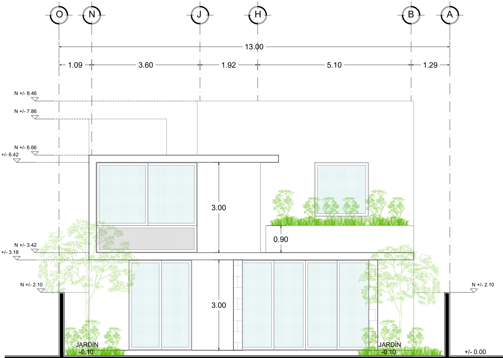
FACHADA SUR
