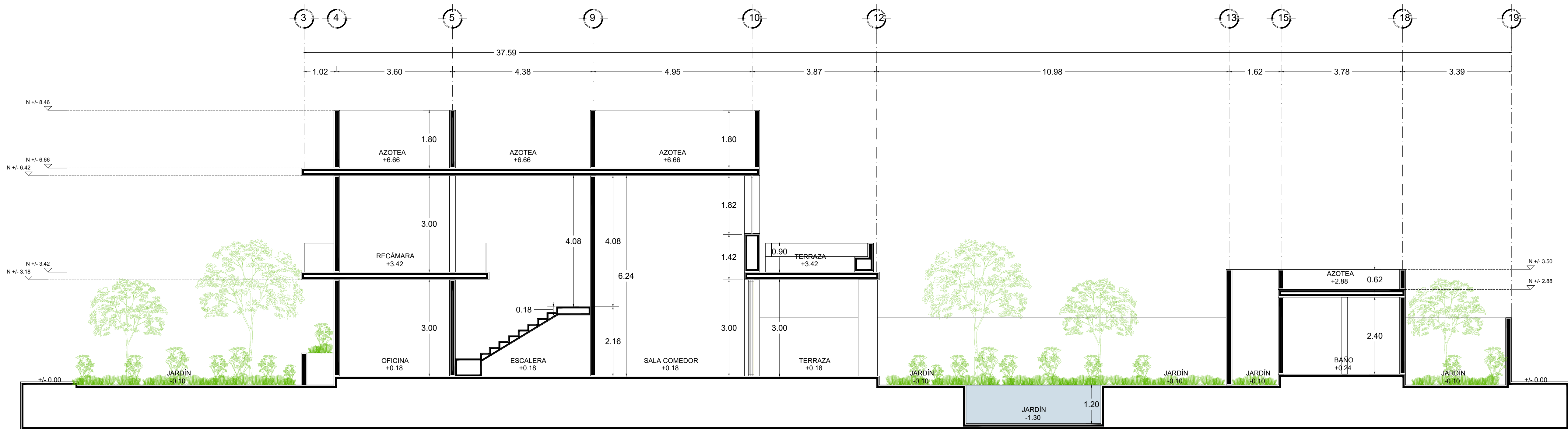
SECCIÓN A
