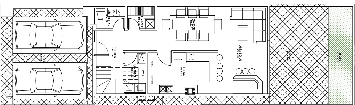
PLANTA BAJA
