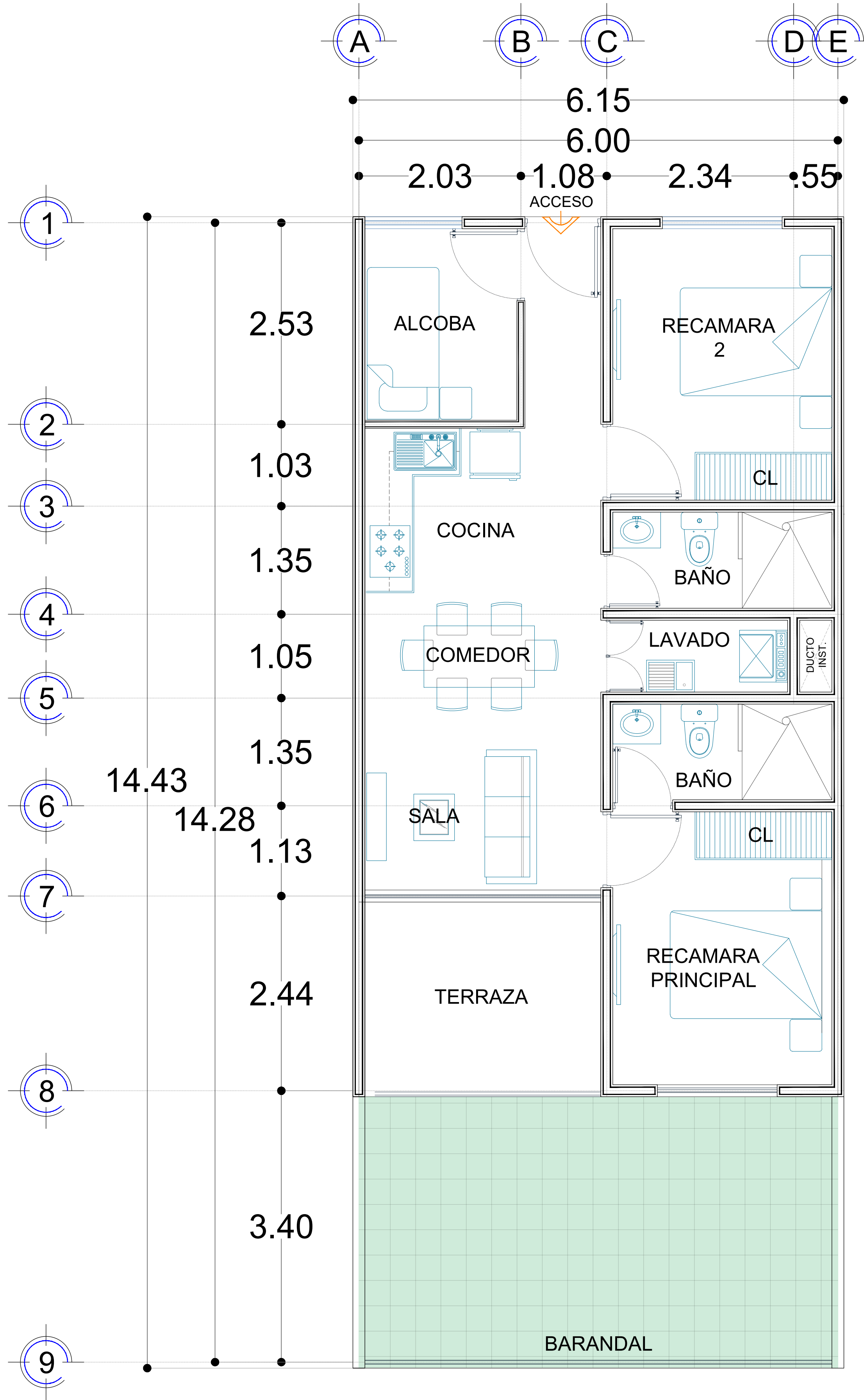
DEPARTAMENTO 2R + ALCOBA PLANTA BAJA
