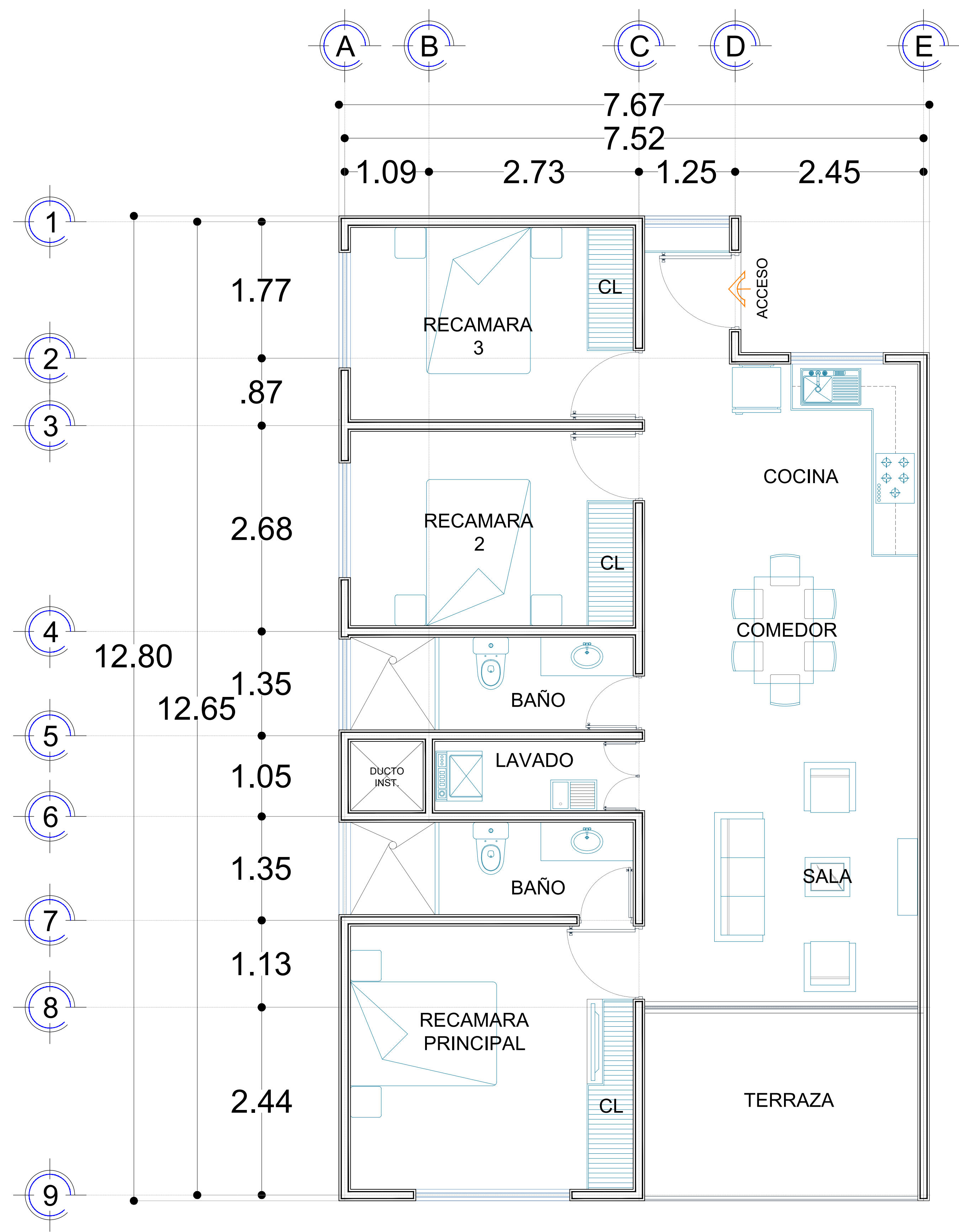
DEPARTAMENTO 3R PISOS DEL NO. 1 AL NO. 9
