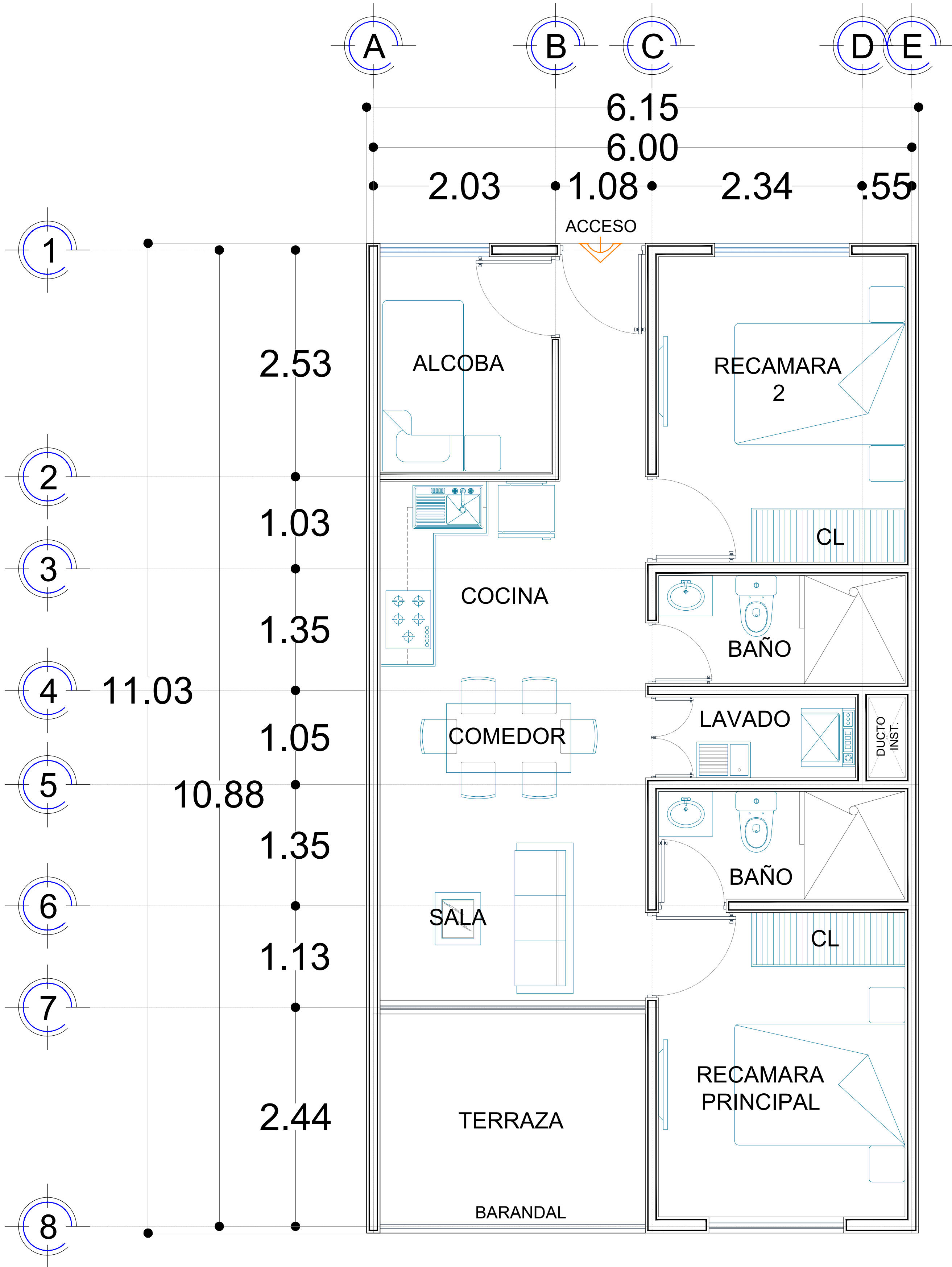
DEPARTAMENTO 2R + ALCOBA PISOS DEL NO. 1 AL NO. 9
