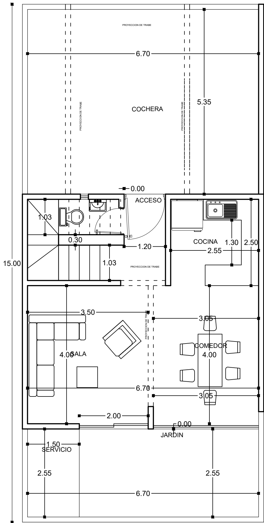
PLANO ARQUITECTONICO PLANTA BAJA 71.42 M2
