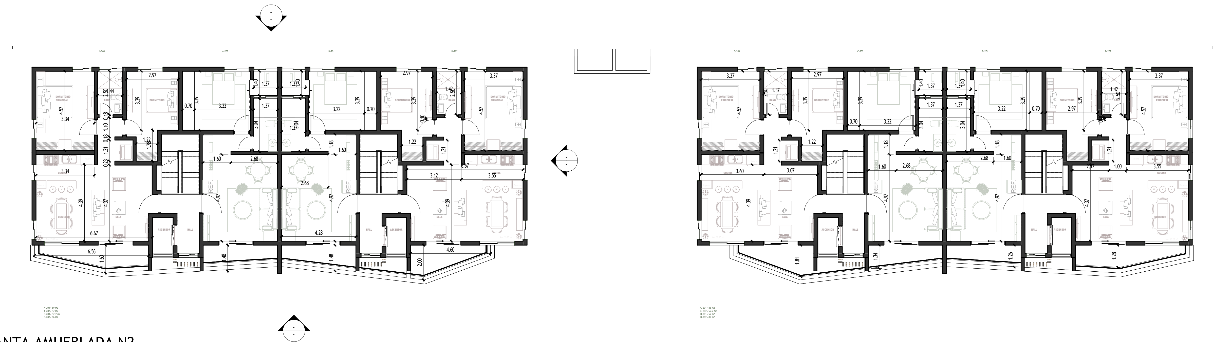
2 PLANTA AMUEBLADA N2 1 : 100
