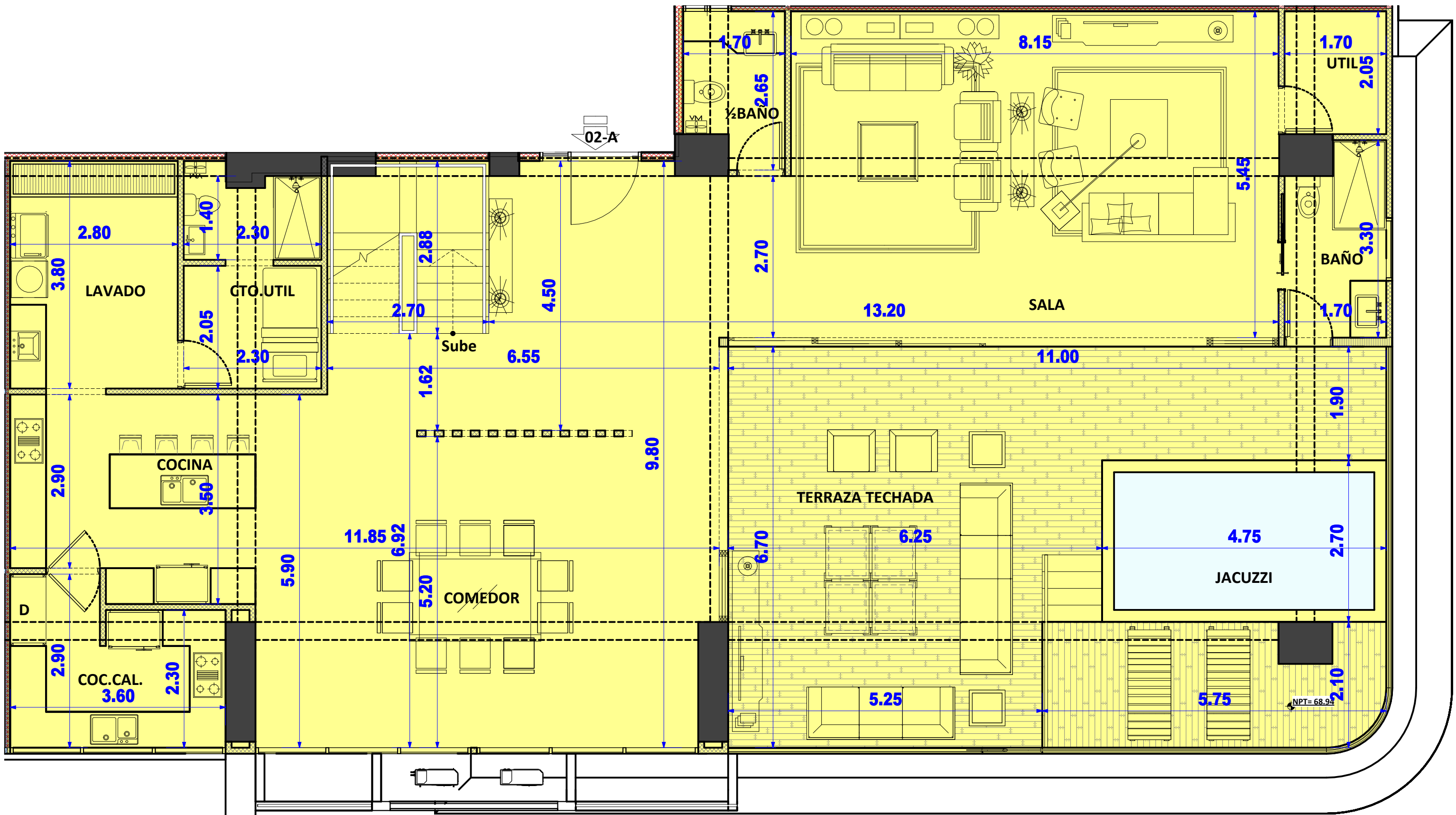
PLANTA BAJA
