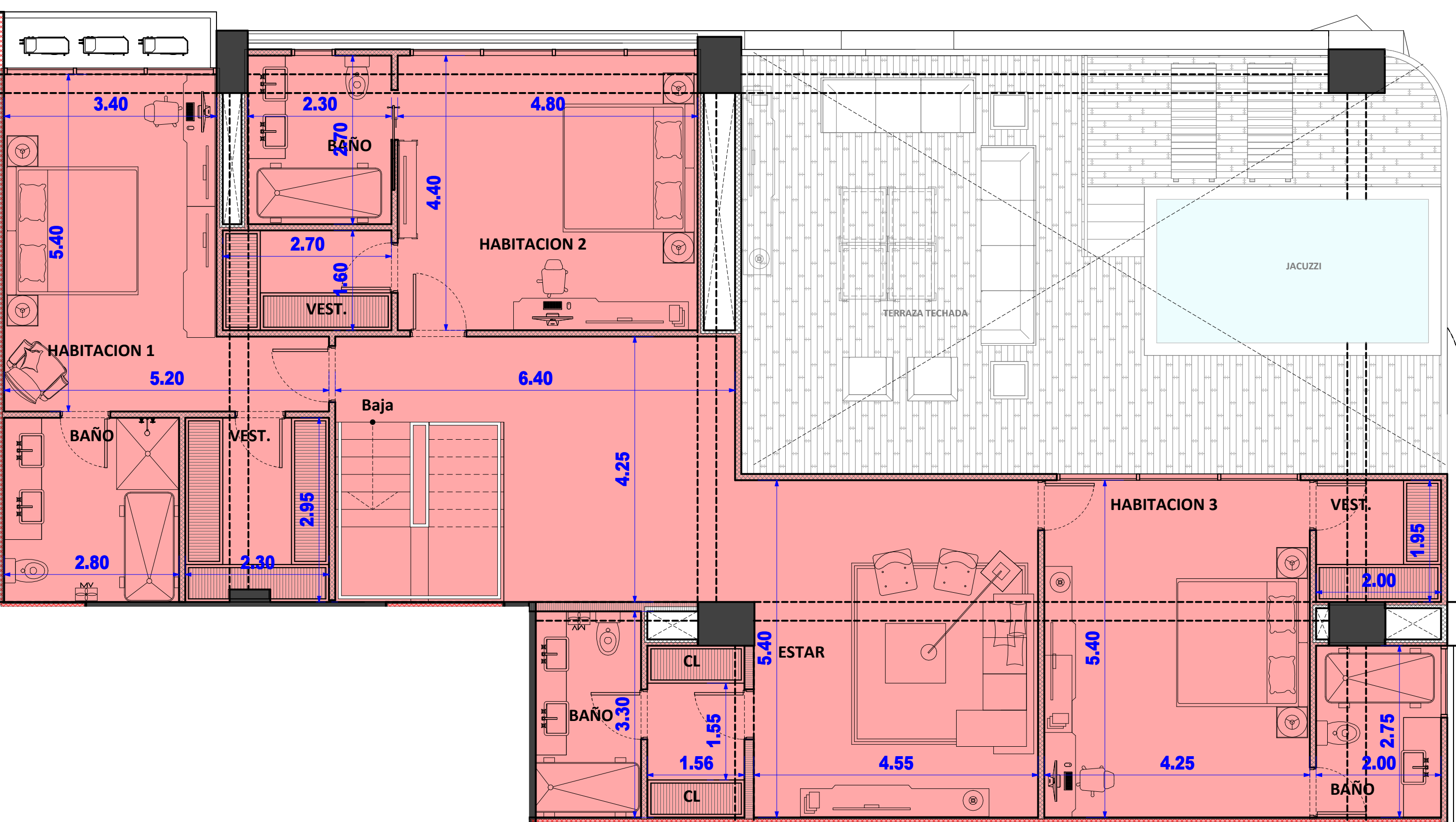
PLANTA ALTA
