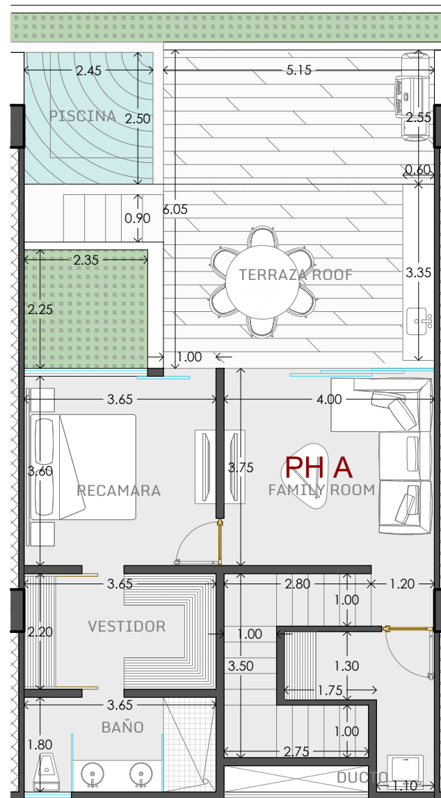
Planta alta
