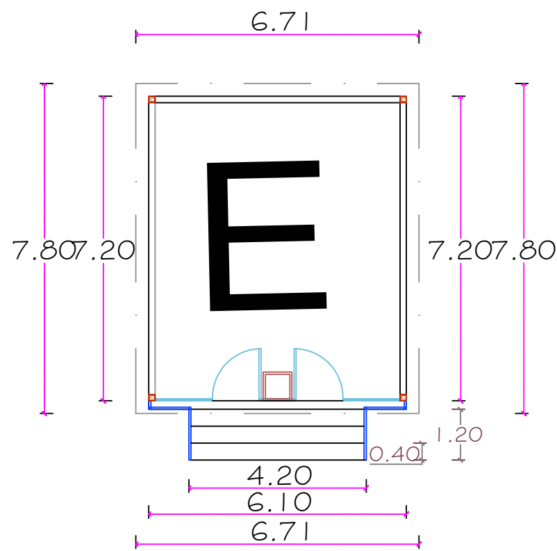
PLANTA Arquitectónica
