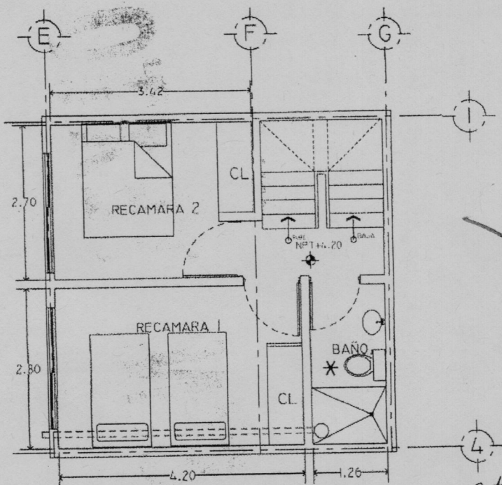
PLANTA PRIMER NIVEL CASA 4 LA QUEMADA 30
