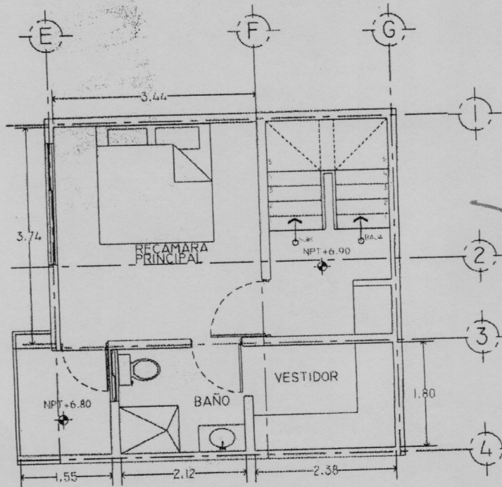
PLANTA SEGUNDO NIVEL CASA 4 LA QUEMADA 30
