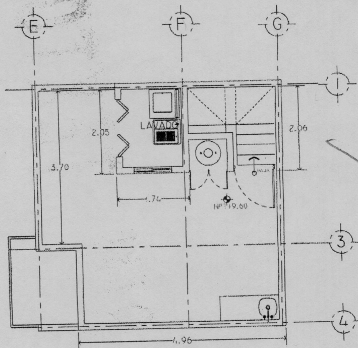
PLANTA AZOTEAS CASA 4 LA QUEMADA 30
