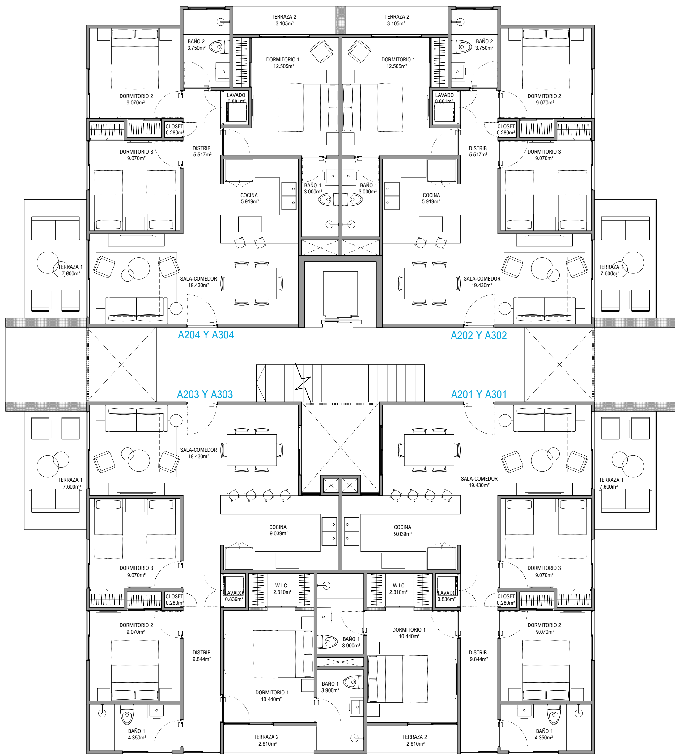
1 NIVELES 2 Y 3 - DISTRIBUCIÓN Y SUPERFICIES E: 1/75
