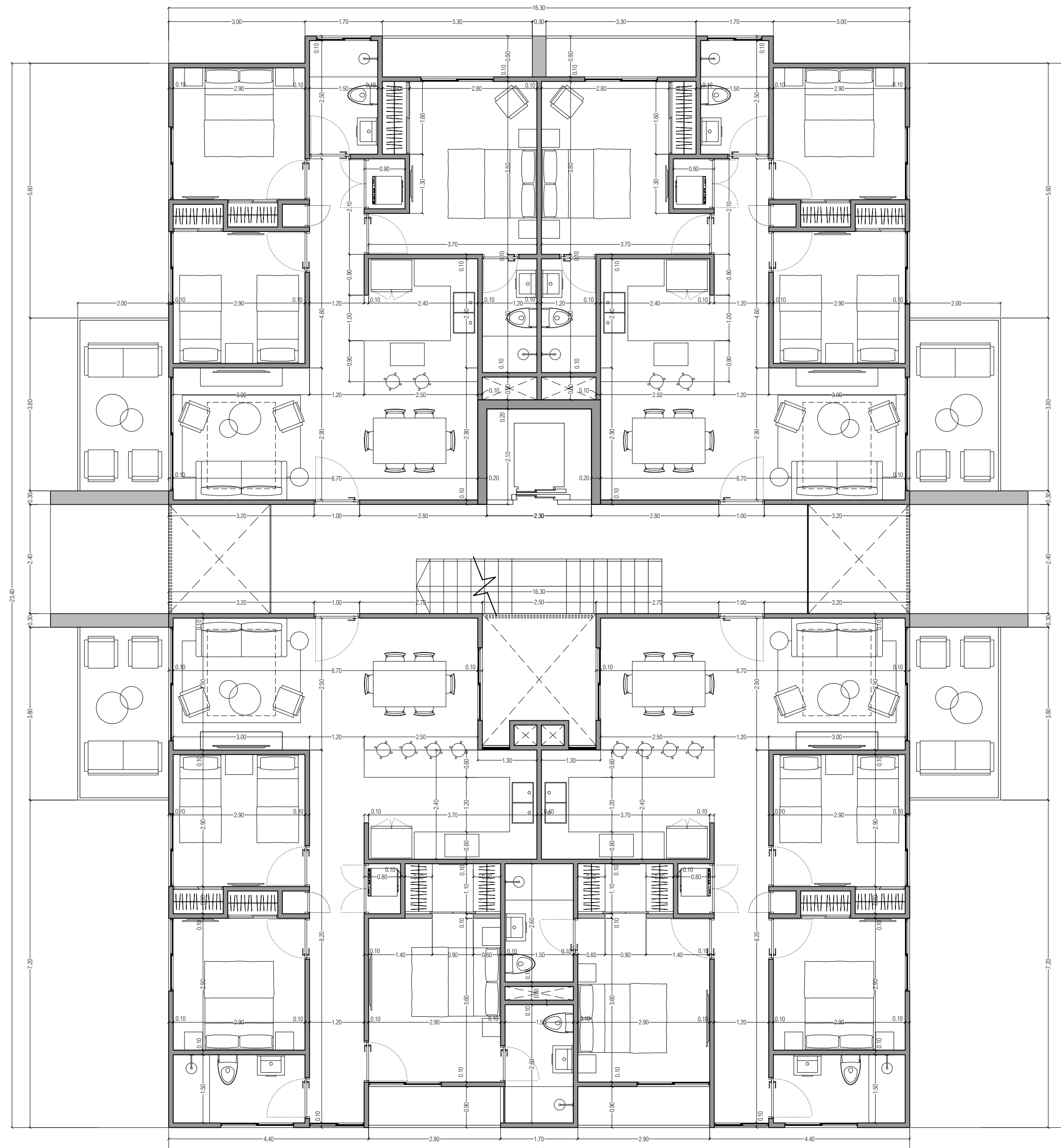
2 NIVELES 2 Y 3 - DIMENSIONES E: 1/75
