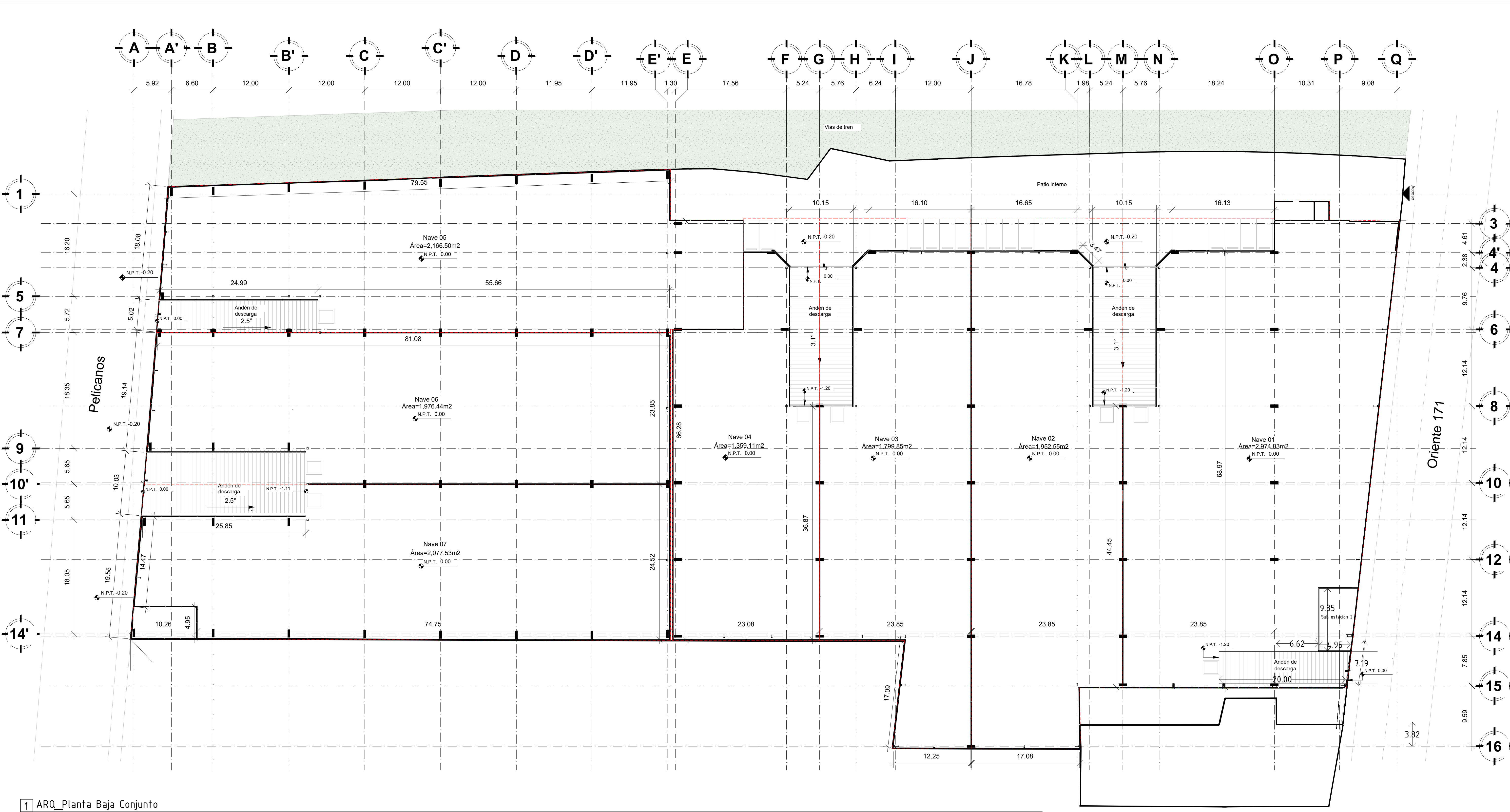
1 ARQ_Planta Baja Conjunto ESC. 1 : 300
