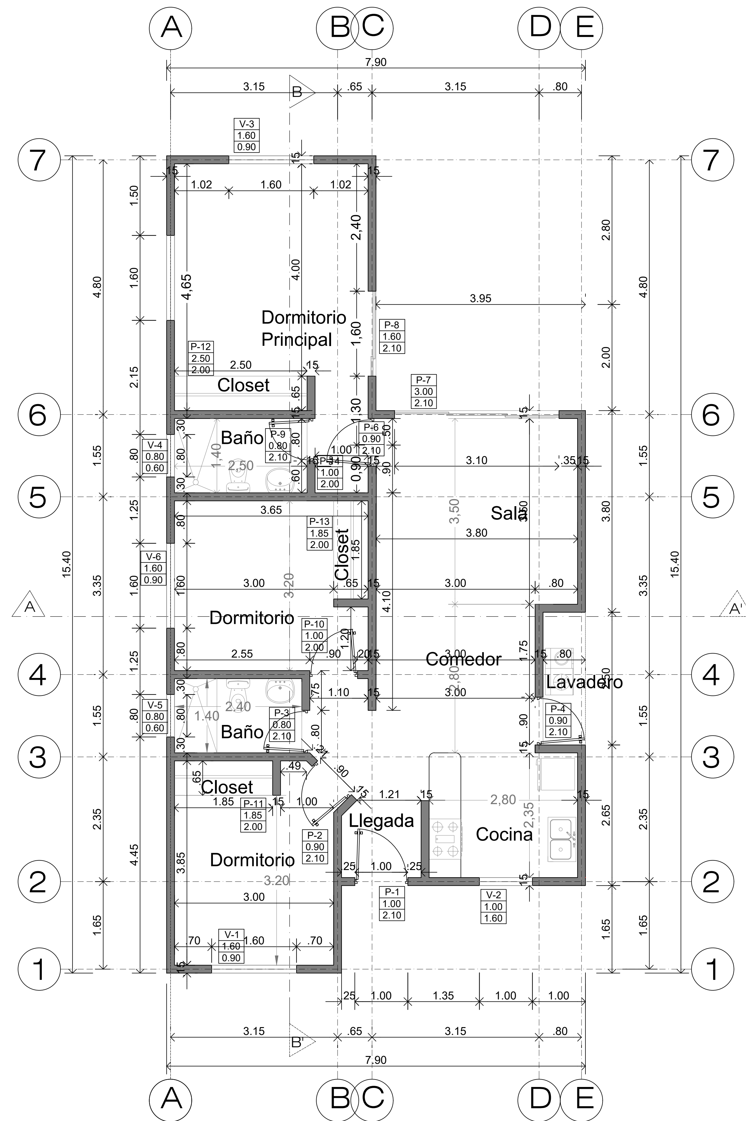
PLANTA DIMENSIONADA VIVIENDA 95 M2 3 HABITACIONES Y 2 BAÑOS
