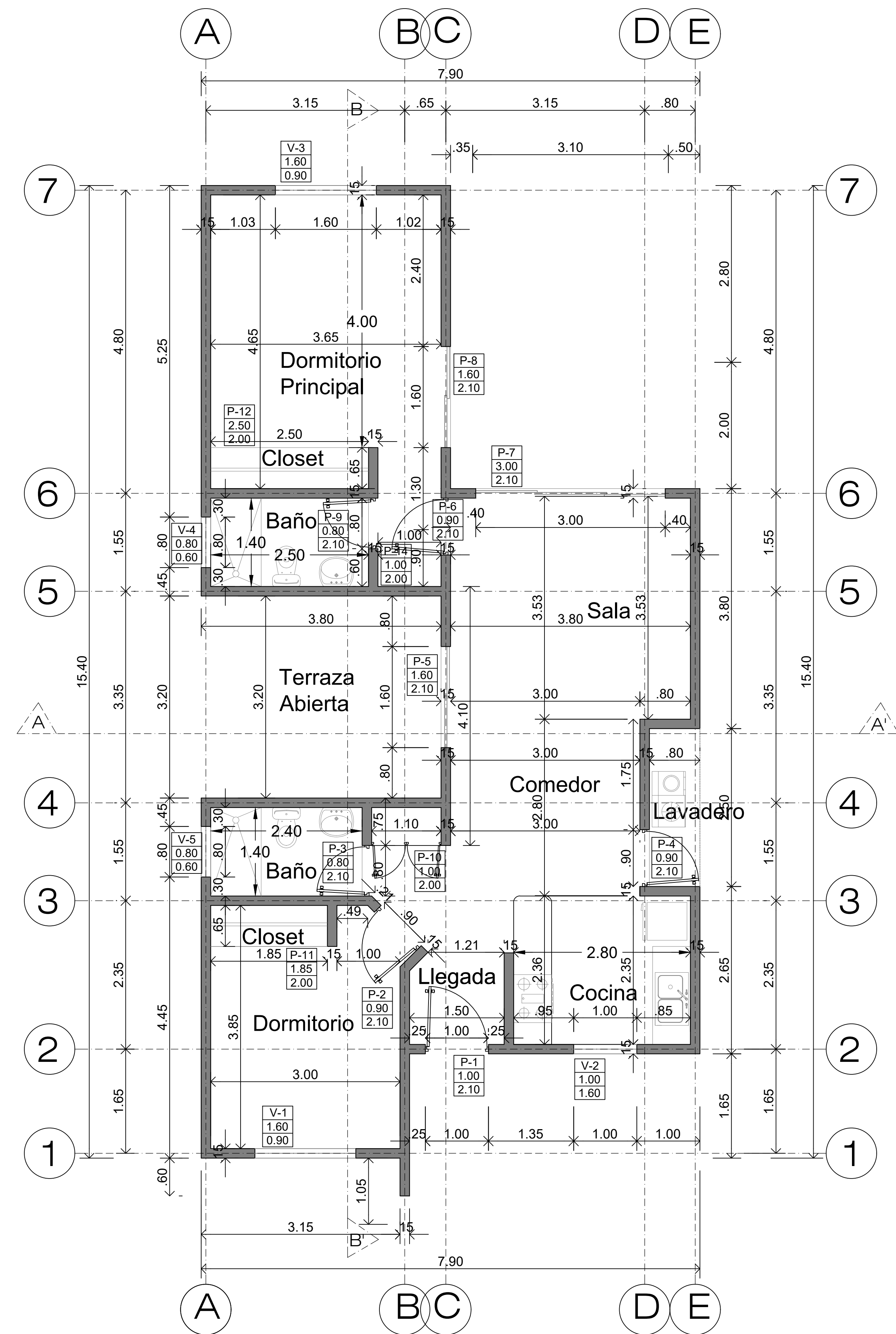
PLANTA DIMENSIONADA VIVIENDA 75 M2 2 HABITACIONES Y 2 BAÑOS
