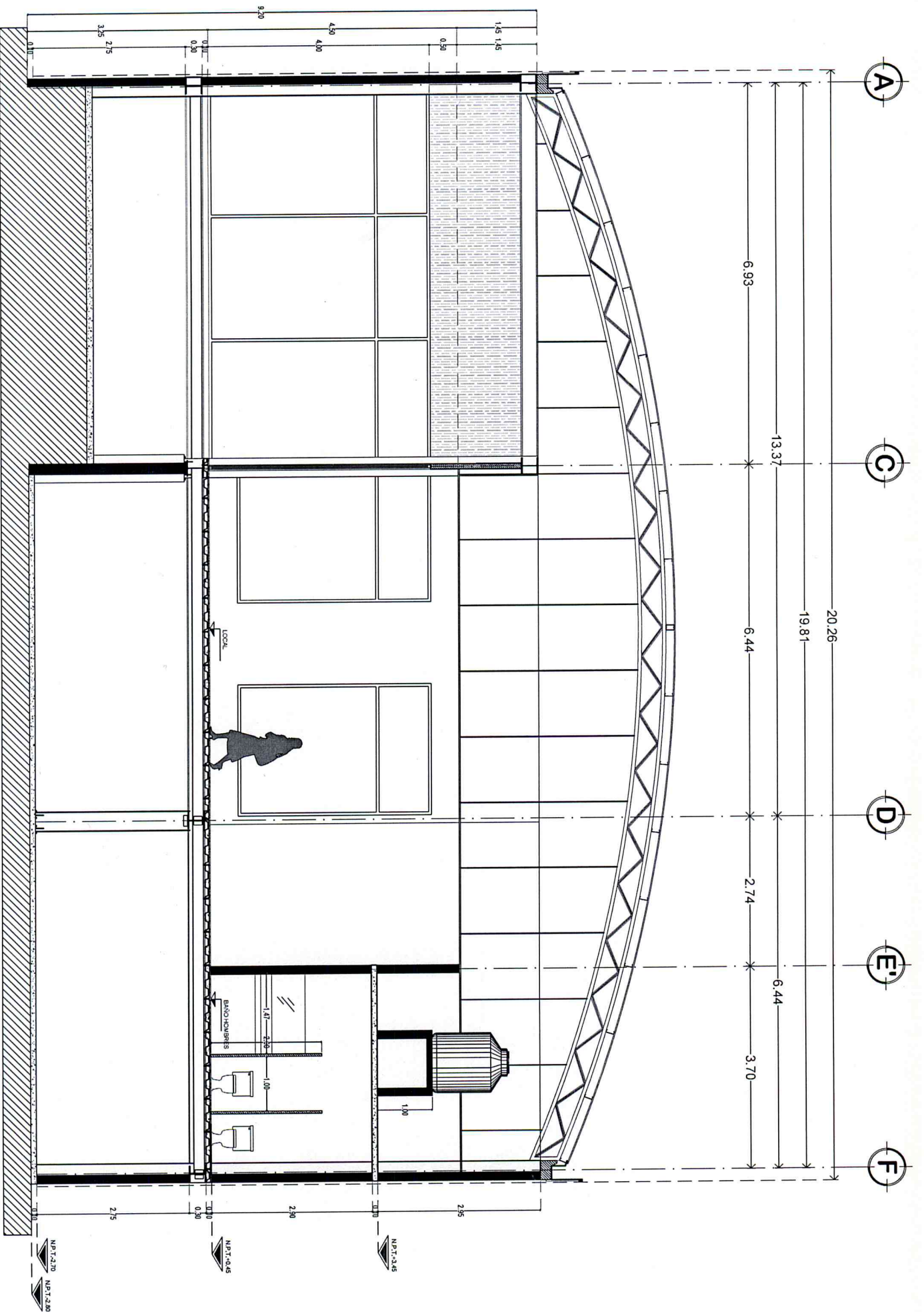
CORTE TRANSVERSAL A-A'
