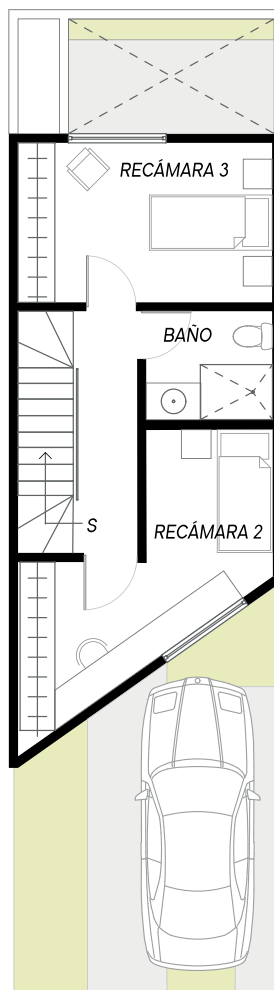
PLANTA NIVEL 1
