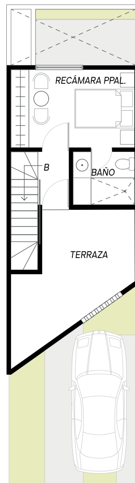
PLANTA NIVEL 2
