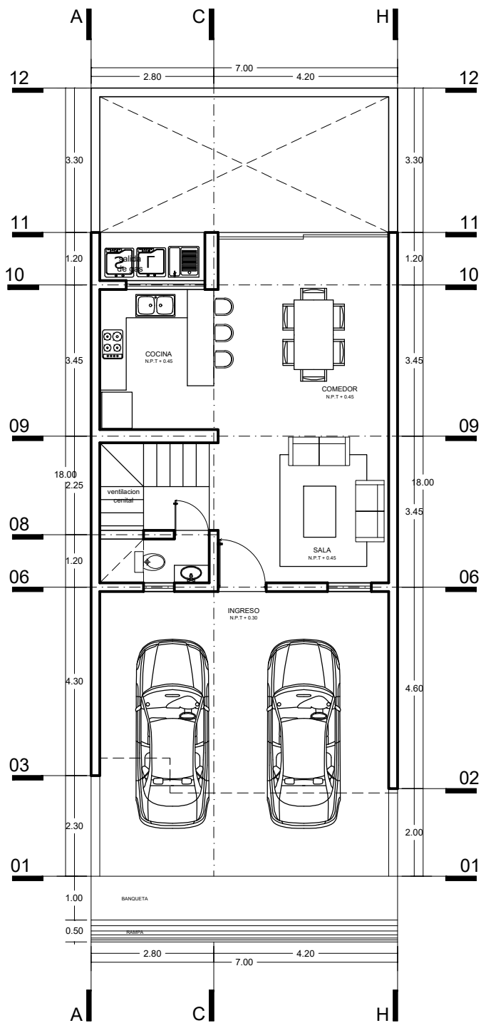
PLANTA ARQUITECTONICA BAJA
