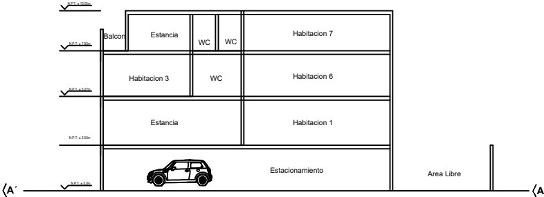
Corte Longitudinal
