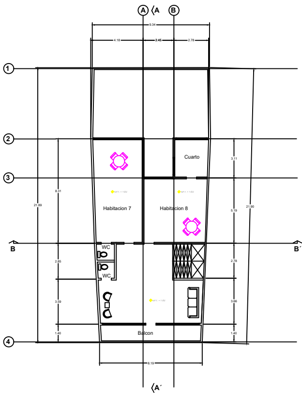
Tercer Piso
