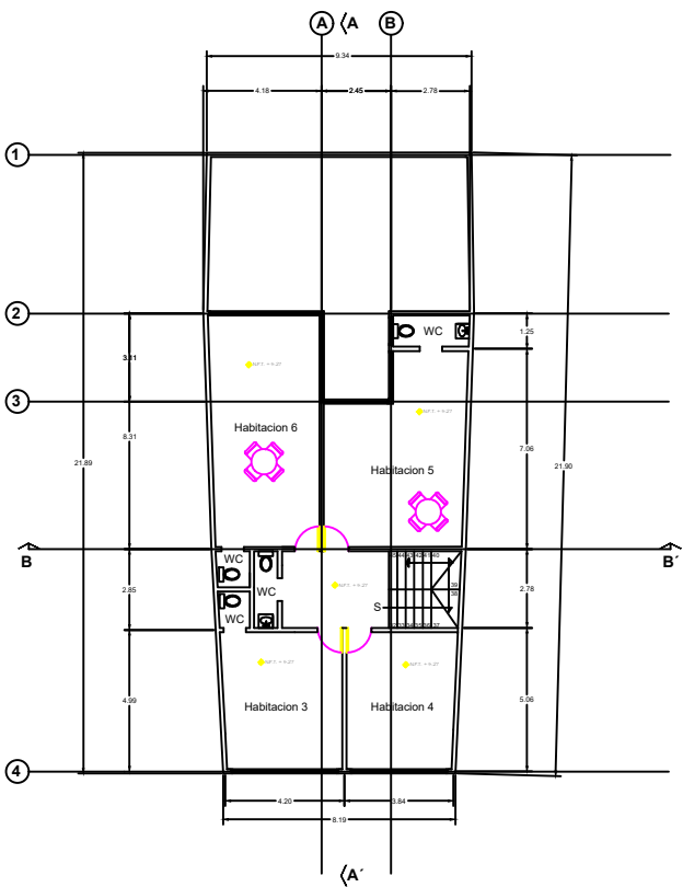
Segundo Piso
