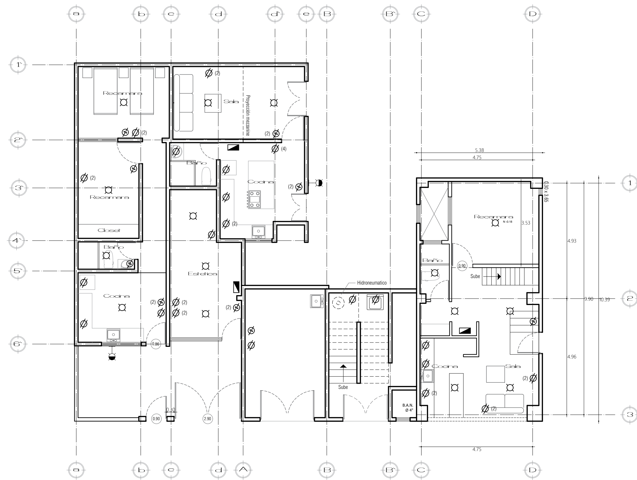
PLANTA BAJA Instalación eléctrica Instalación Hdo - Sanitaria
