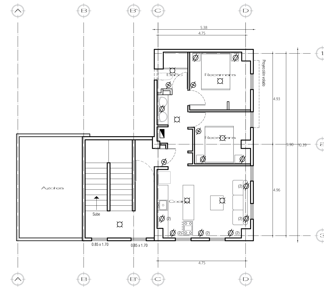
PLANTA 2do NIVEL Instalación eléctrica Instalación Hdo - Sanitaria
