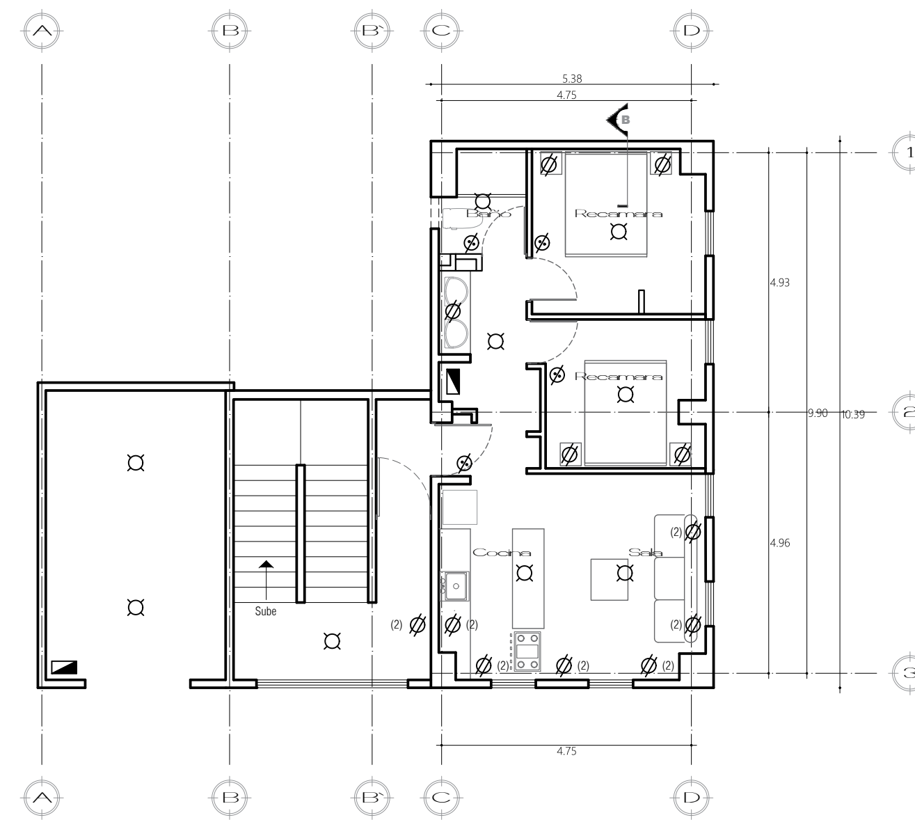
PLANTA 1er NIVEL Instalación eléctrica Instalación Hdo - Sanitaria
