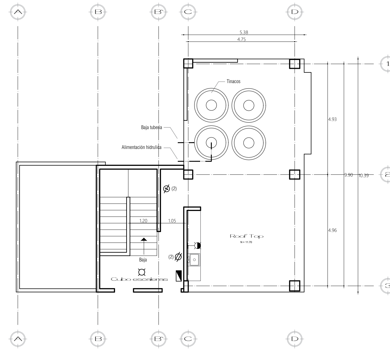
PLANTA 3er NIVEL Instalación eléctrica Instalación Hdo - Sanitaria
