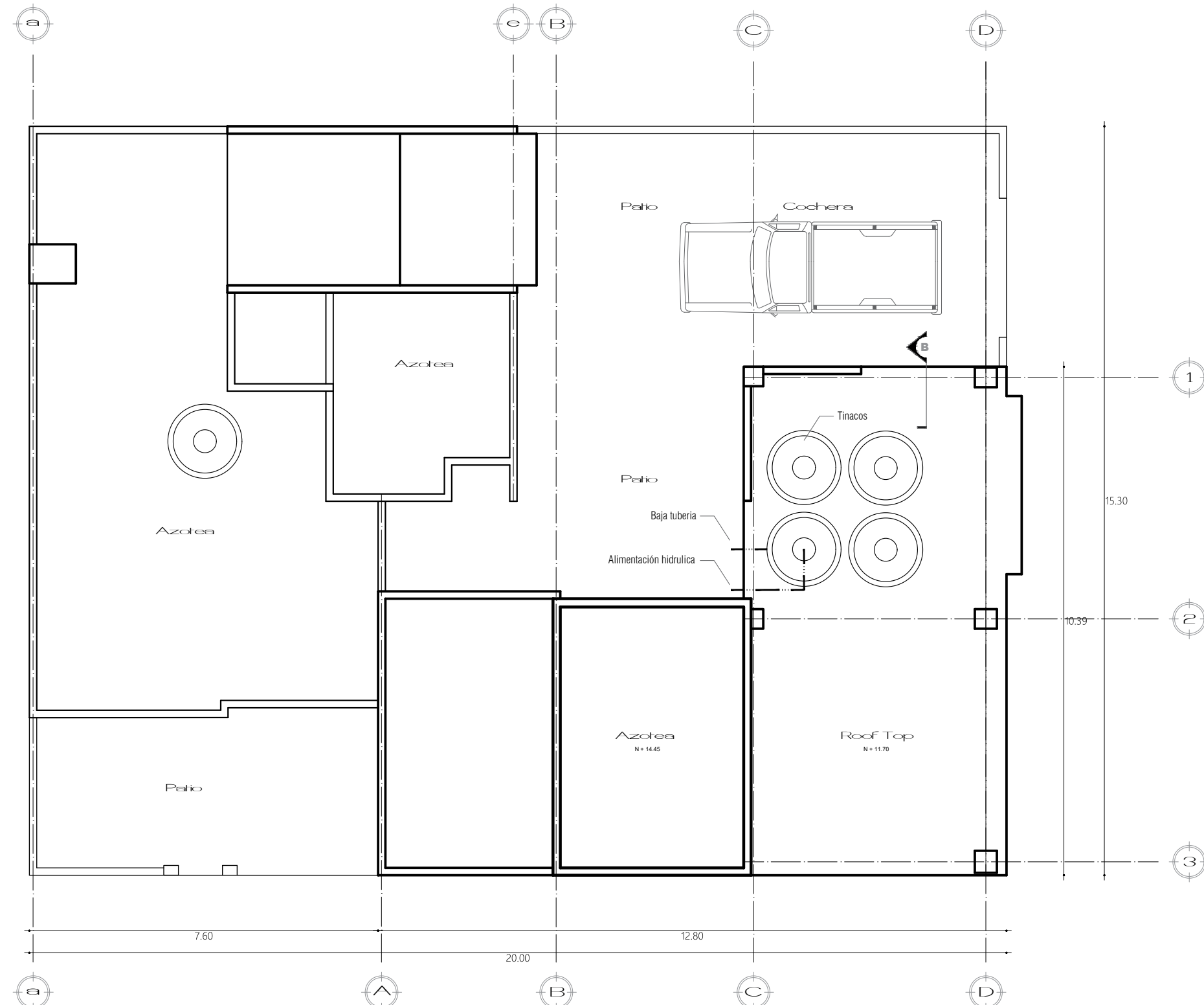
PLANTA DE CUCHITRIL Instalación Hdo - Sanitaria
