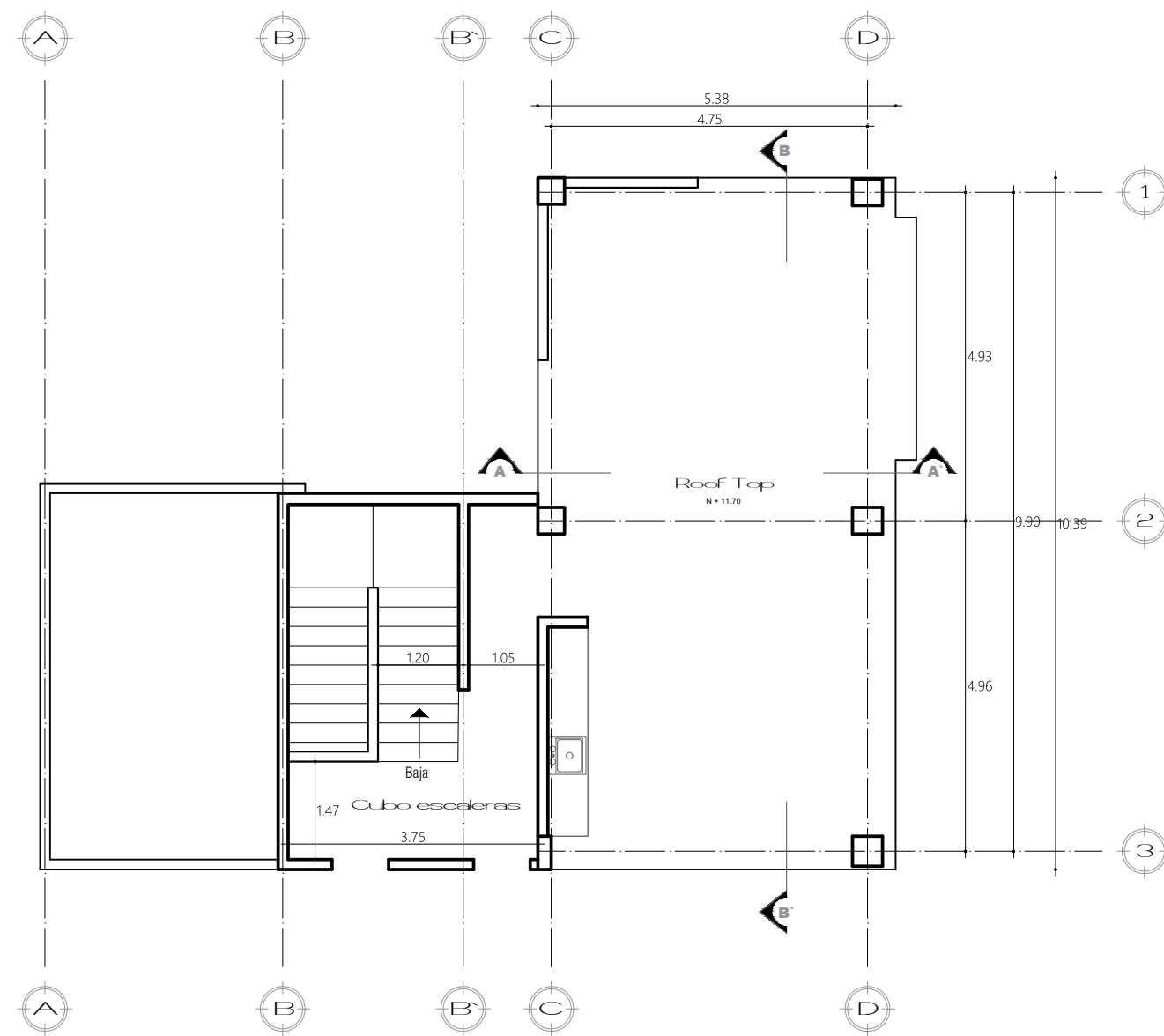
PLANTA 3er NIVEL
