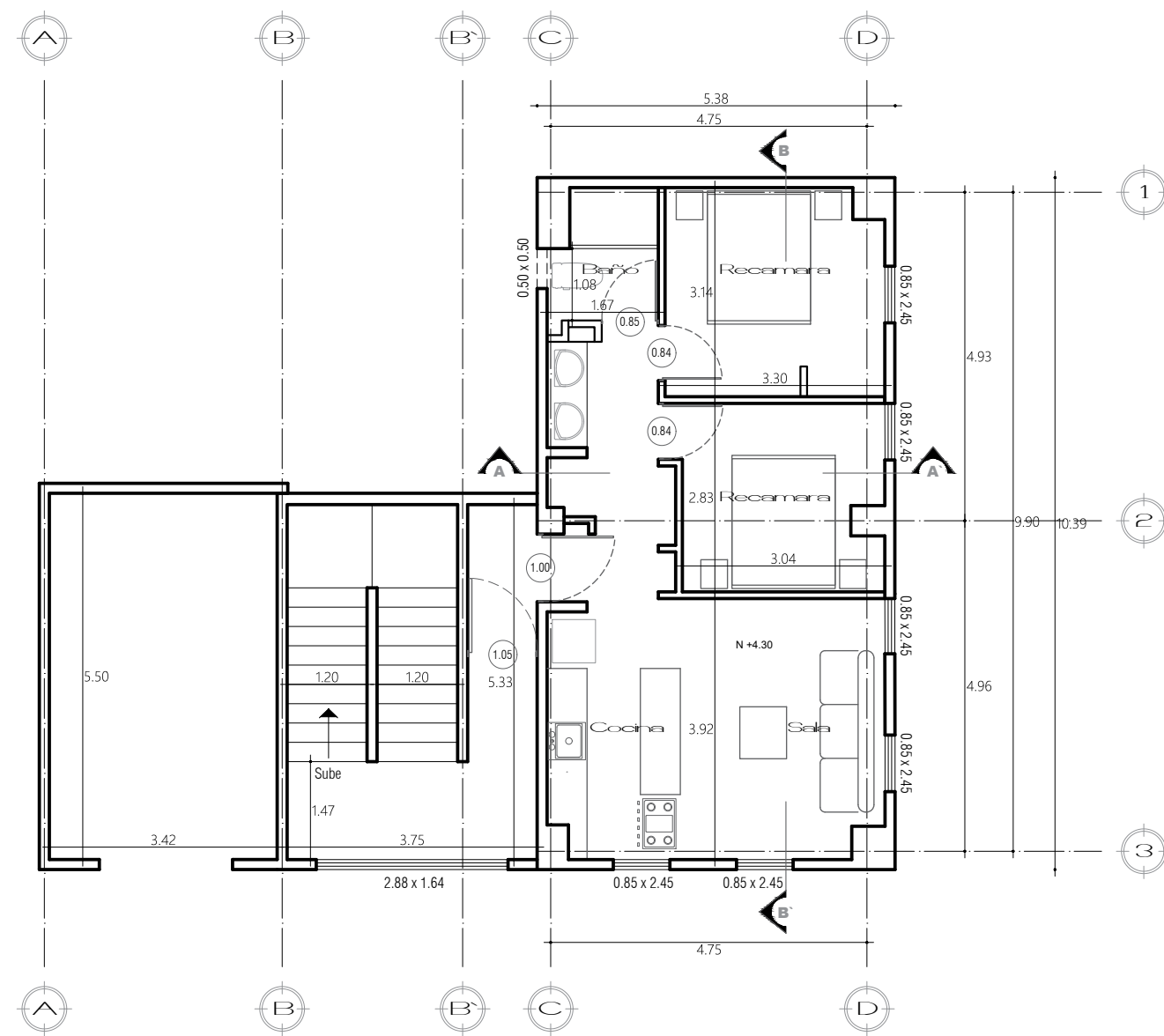
PLANTA 1er NIVEL
