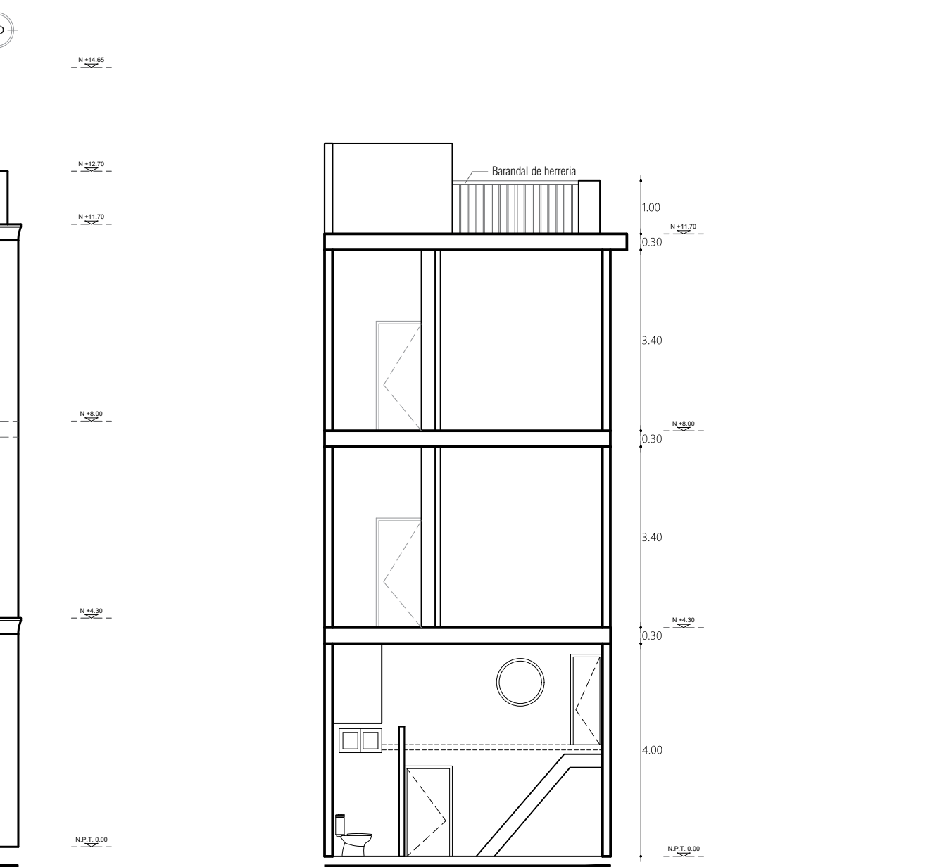
CORTE A-A
