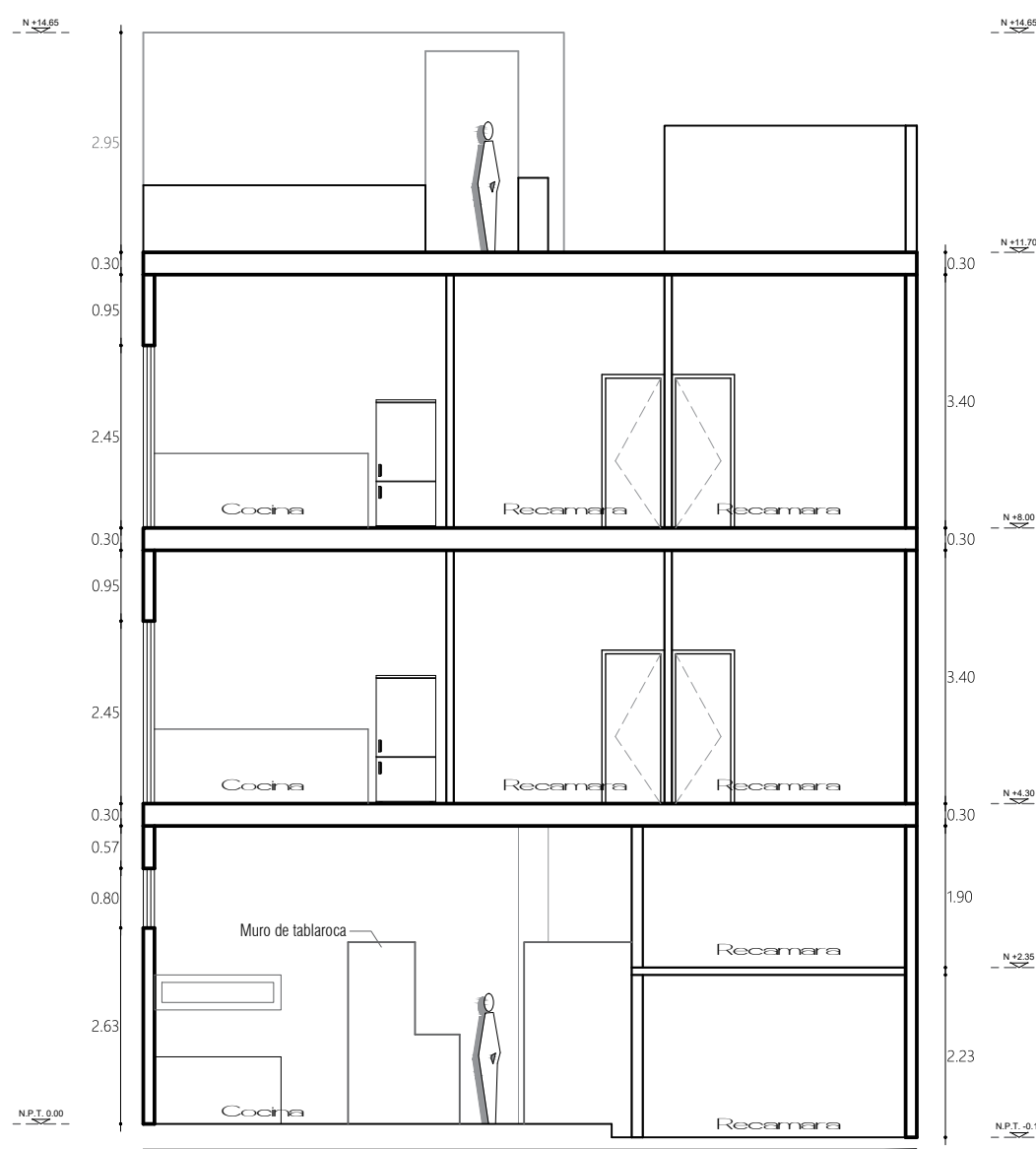
CORTE B-B
