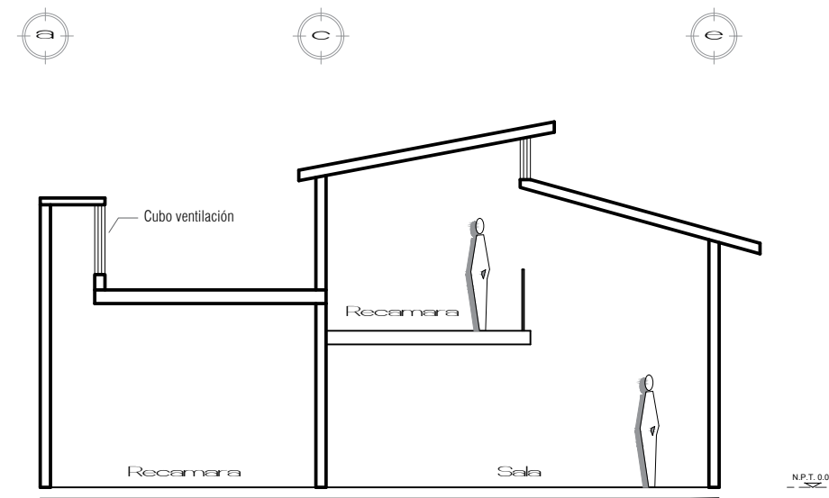
CORTE X-X
