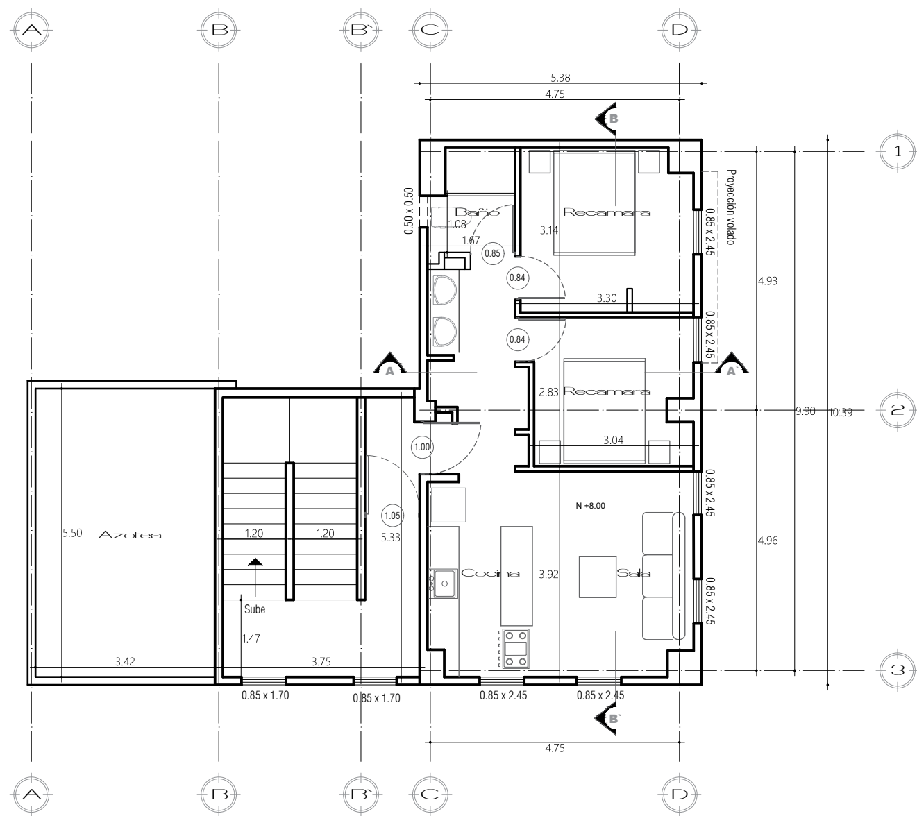
PLANTA 2do NIVEL
