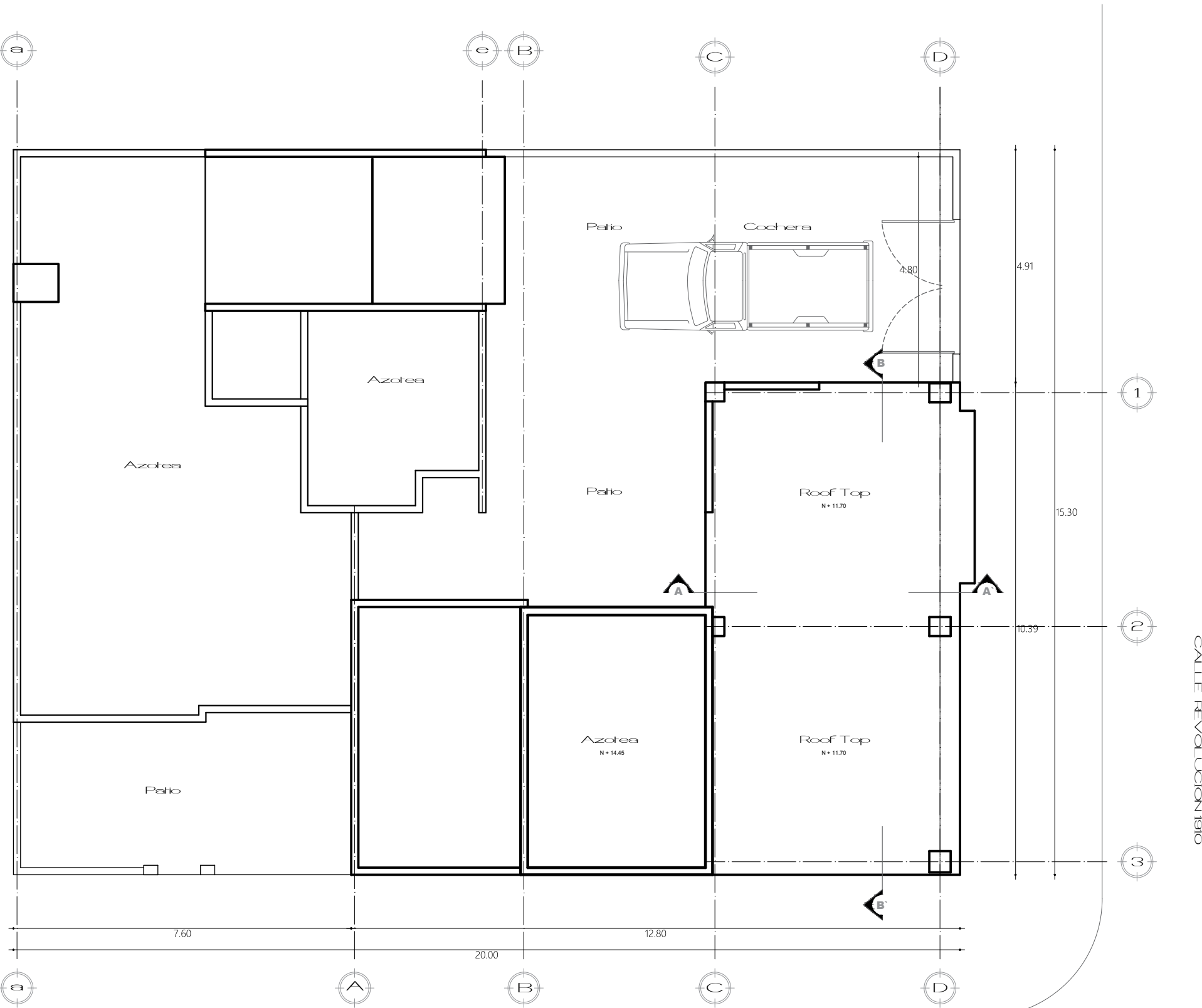
PLANTA DE CONJUNTO
