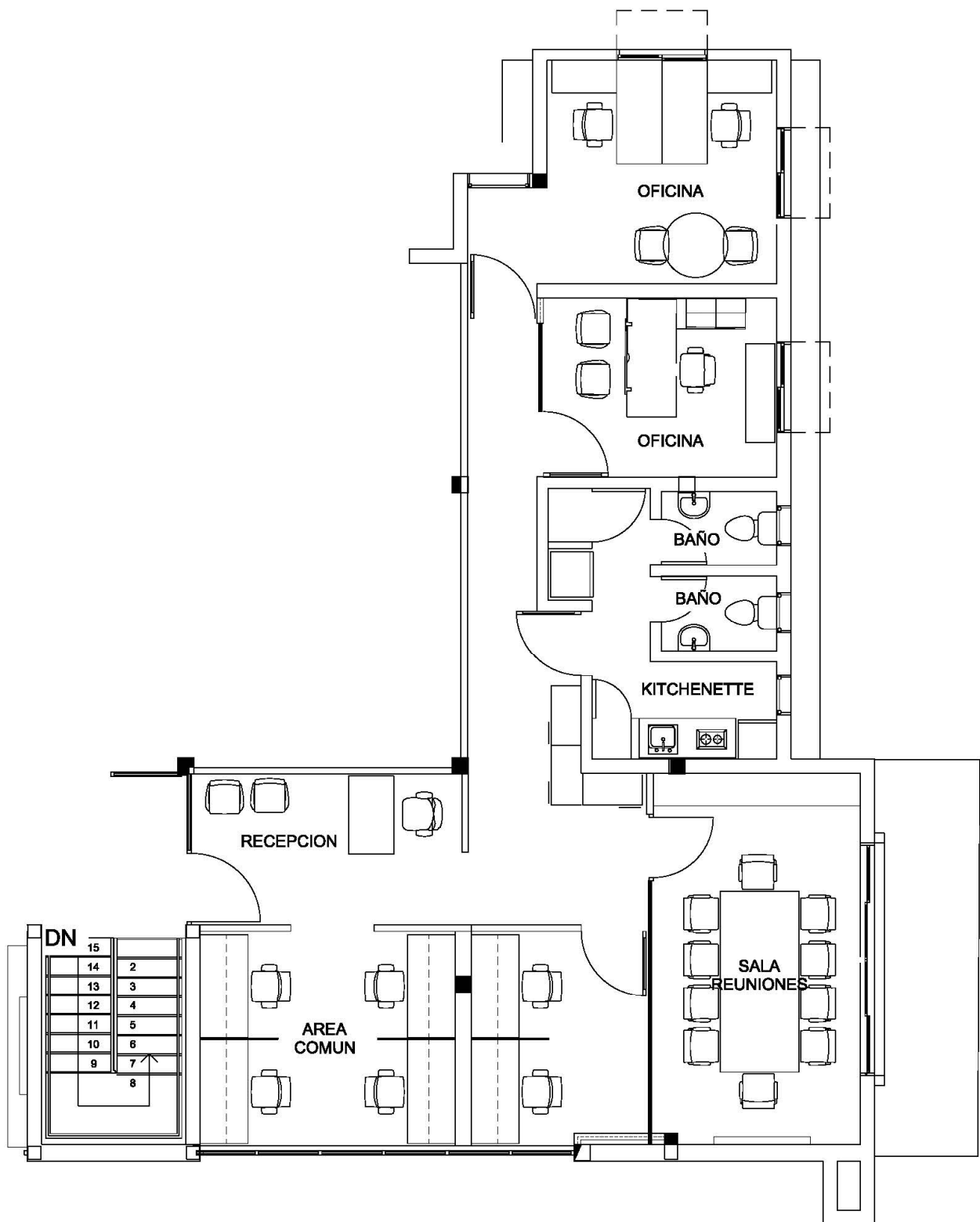
PLANTA - 120m2
