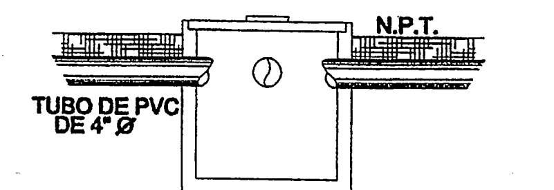
DETALLE DE REGISTRO
