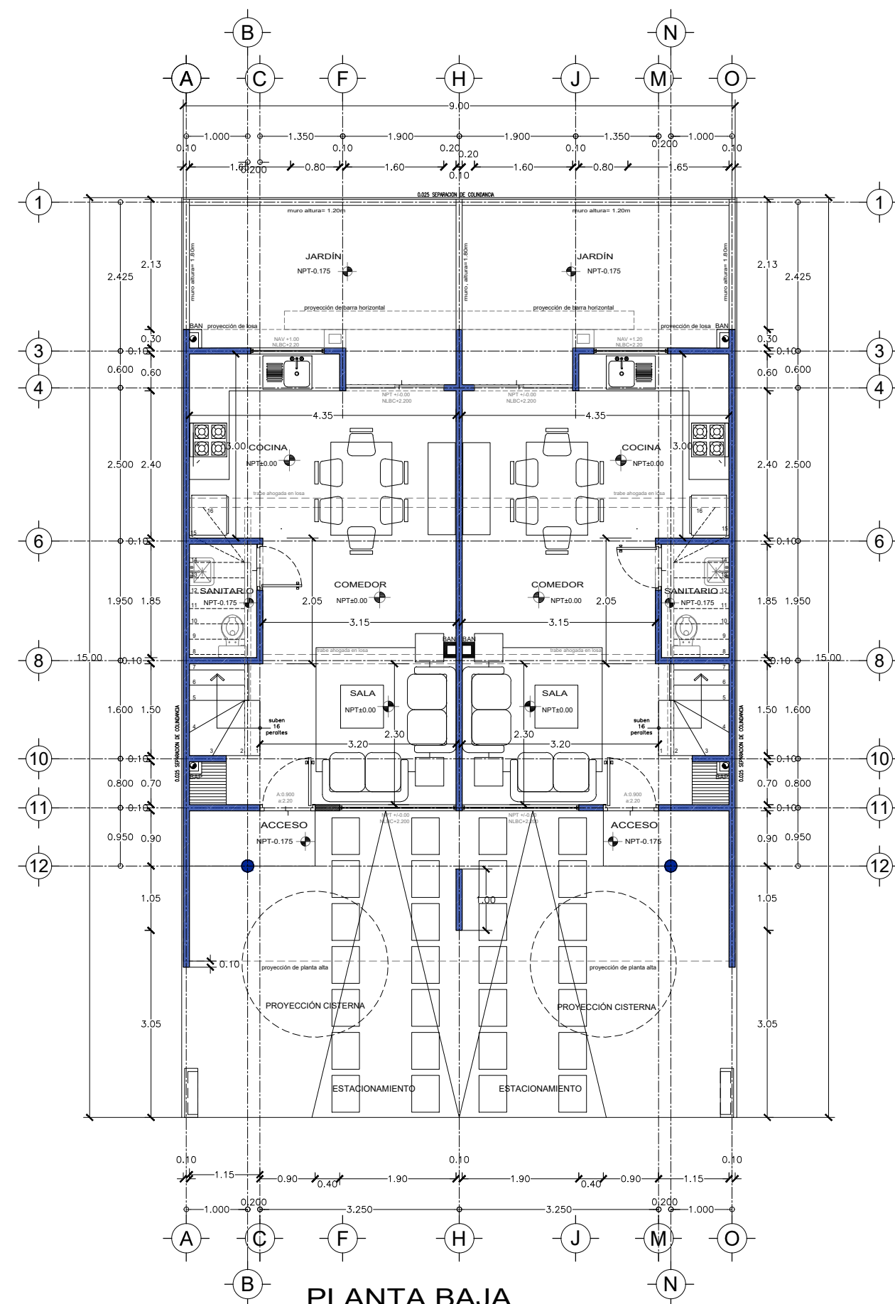
PLANTA BAJA
