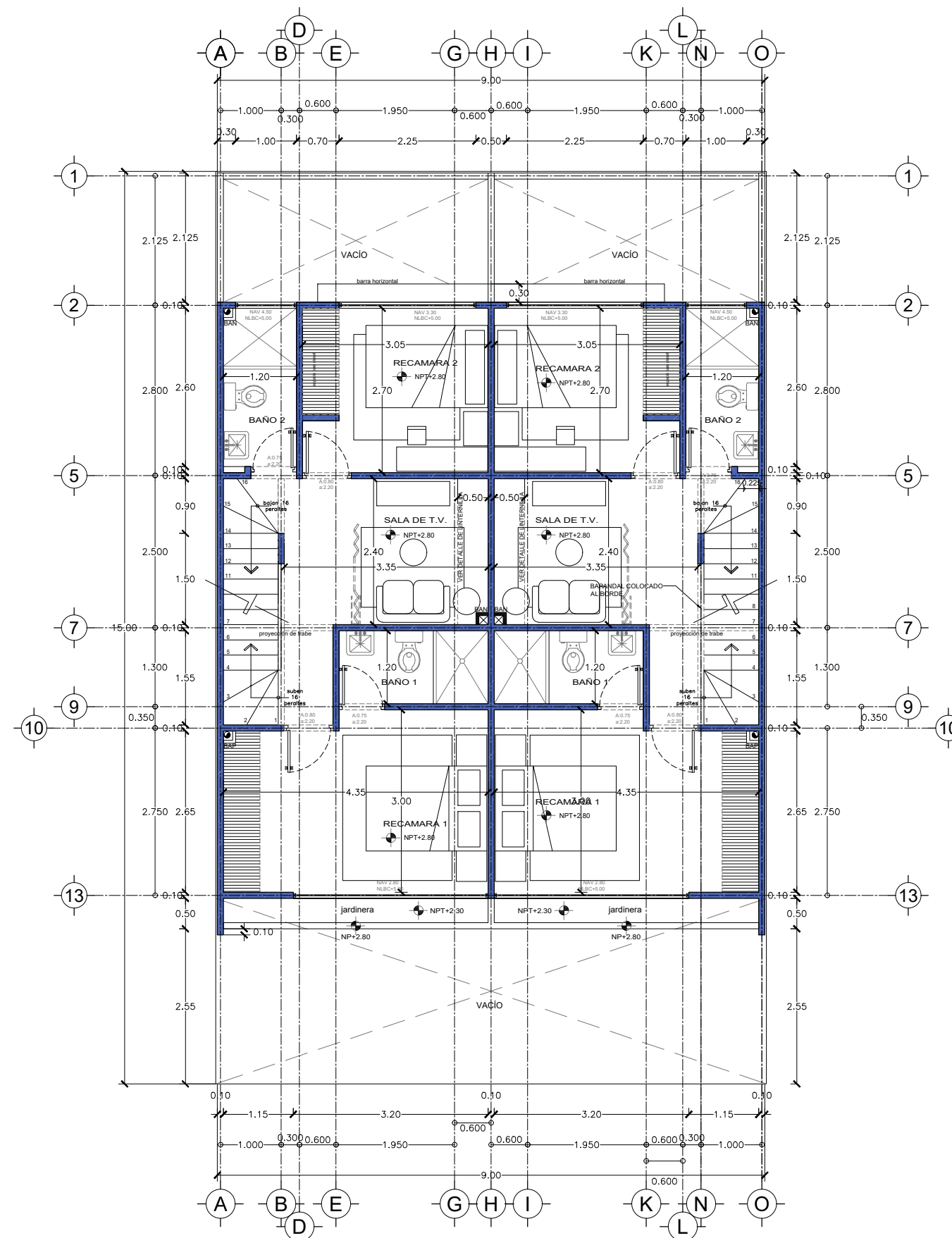
PLANTA ALTA
