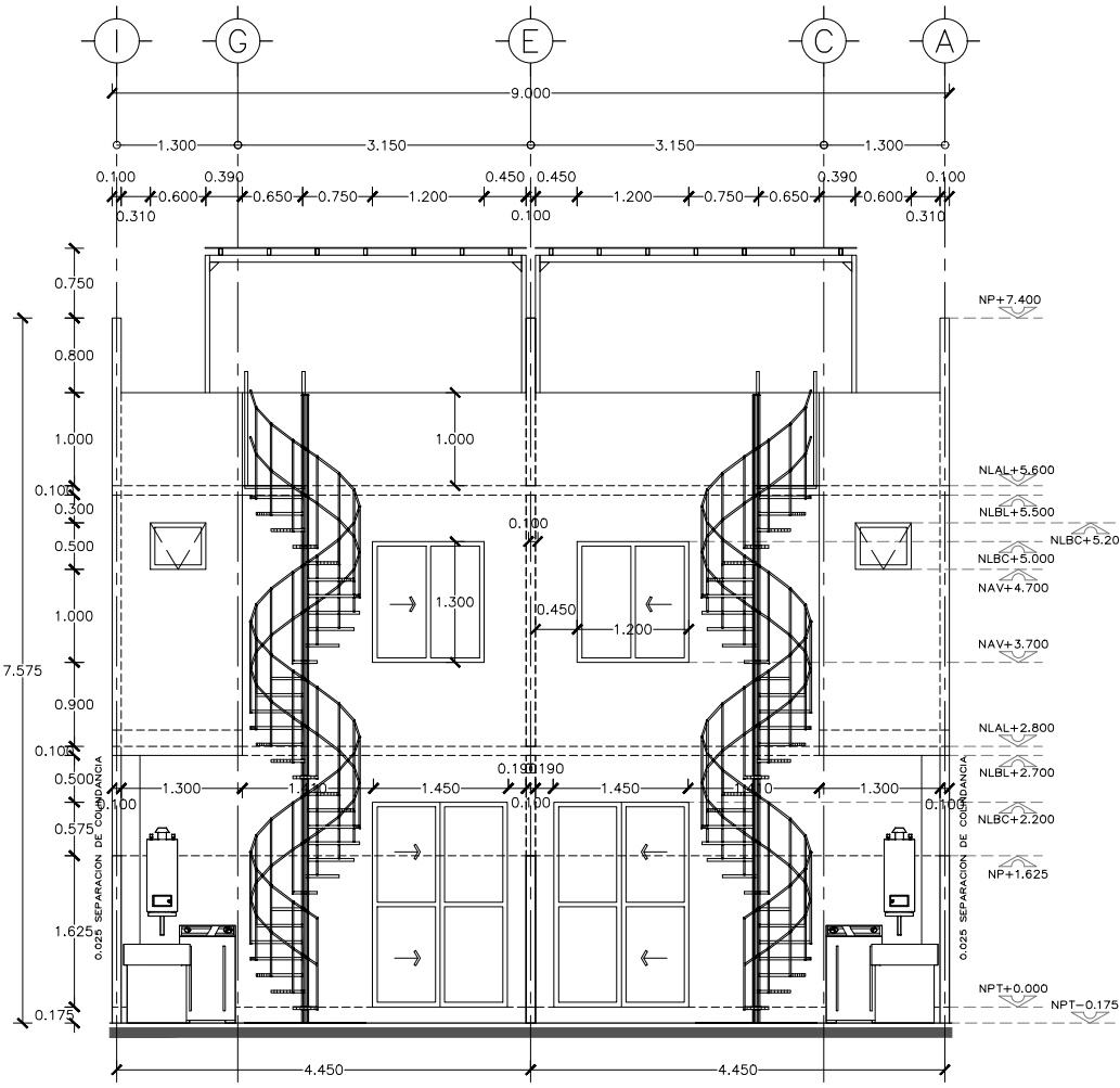
FACHADA POSTERIOR
