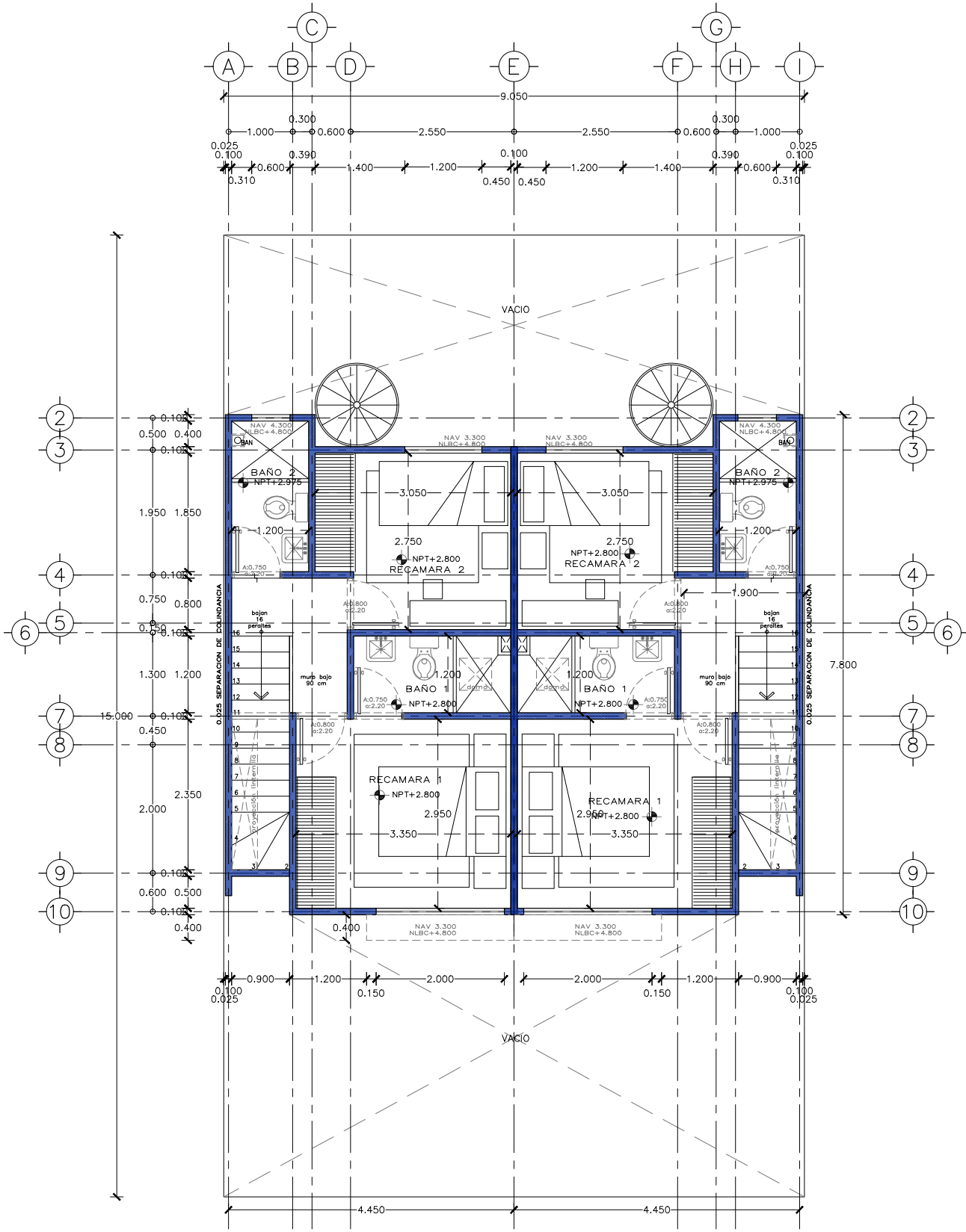
PLANTA ALTA
