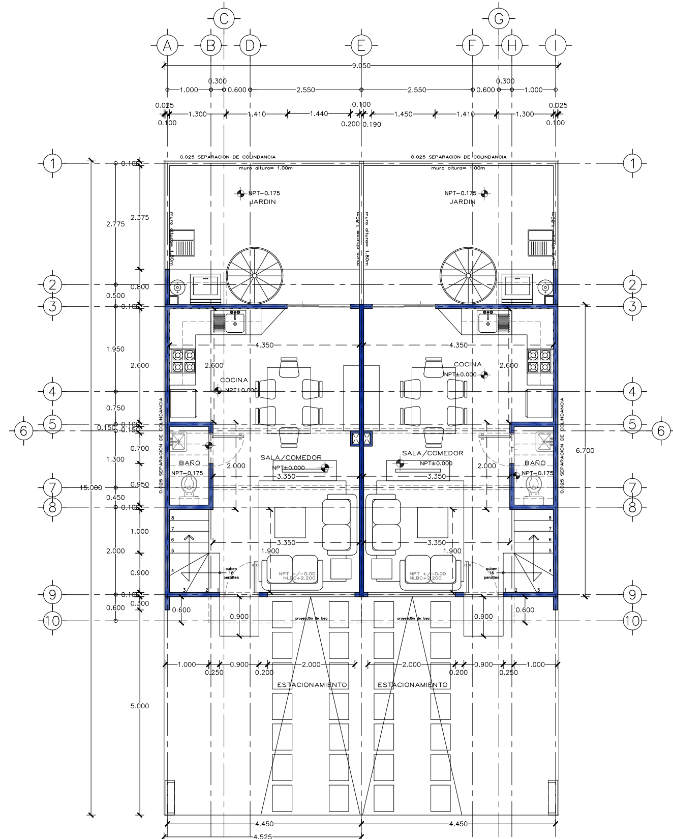
PLANTA BAJA
