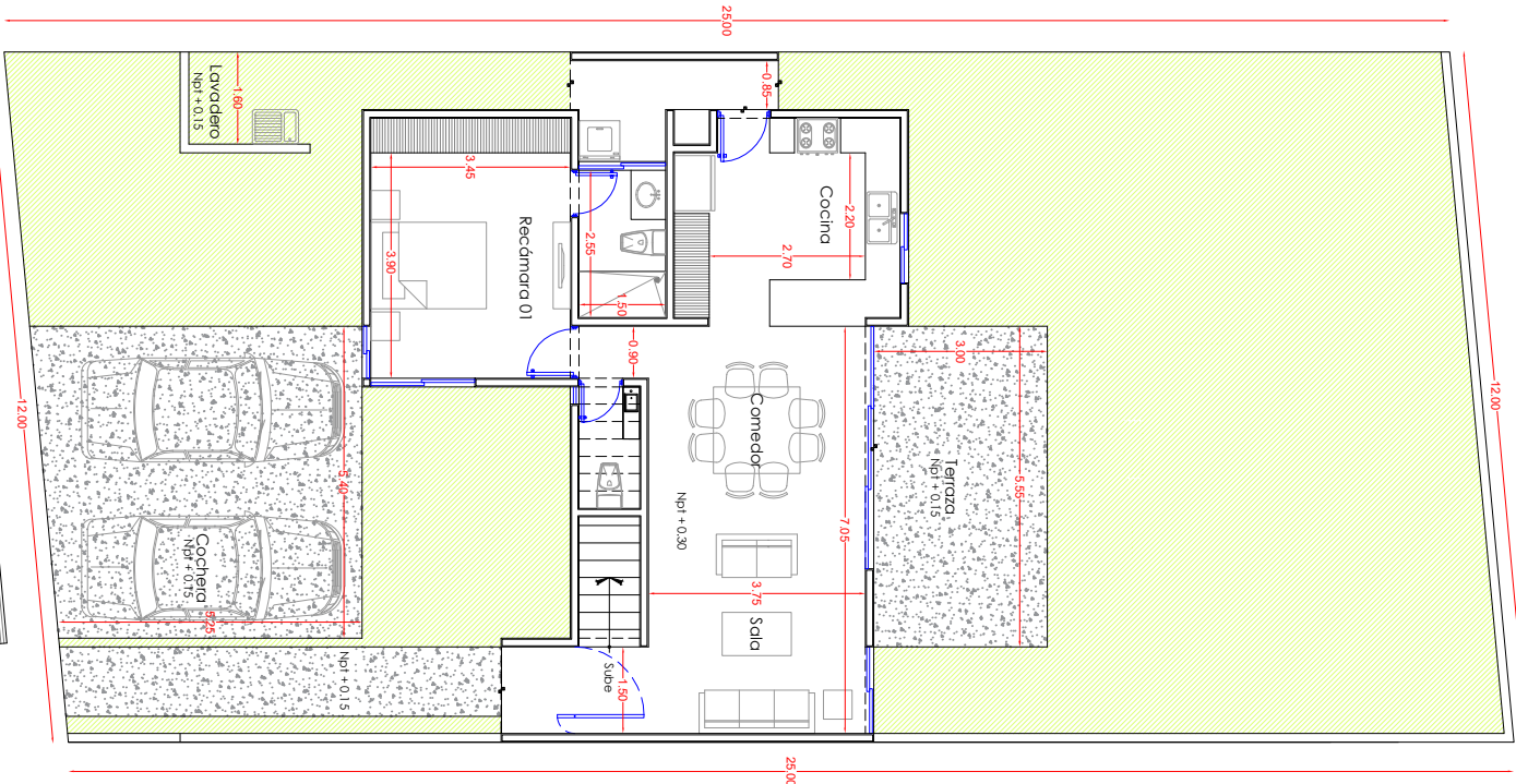
PLANTA BAJA
