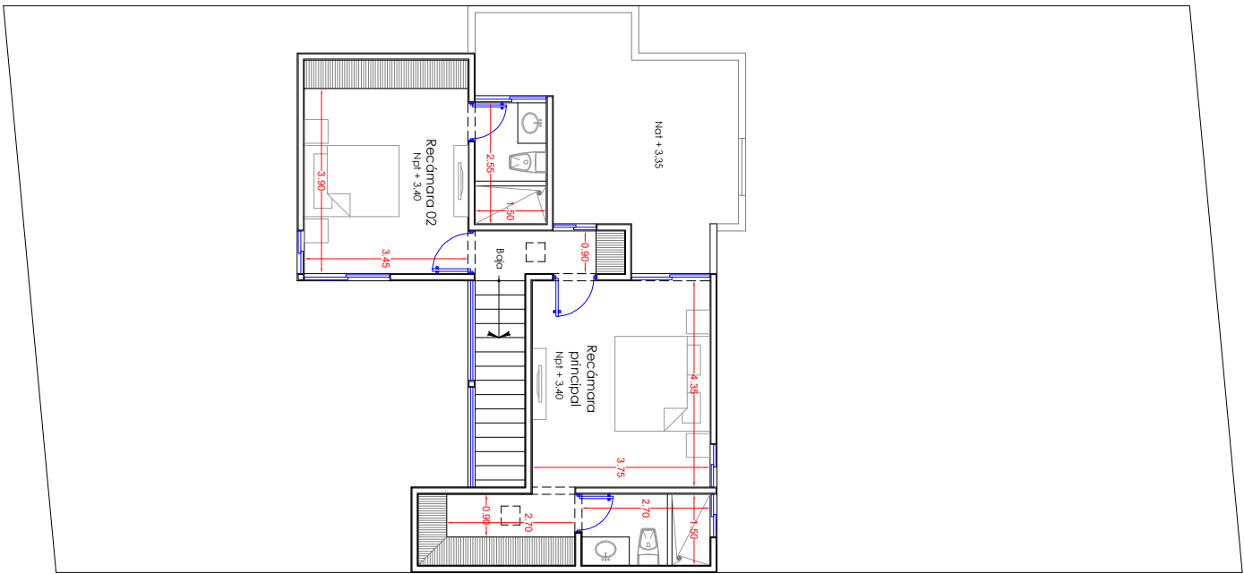
PLANTA ALTA
