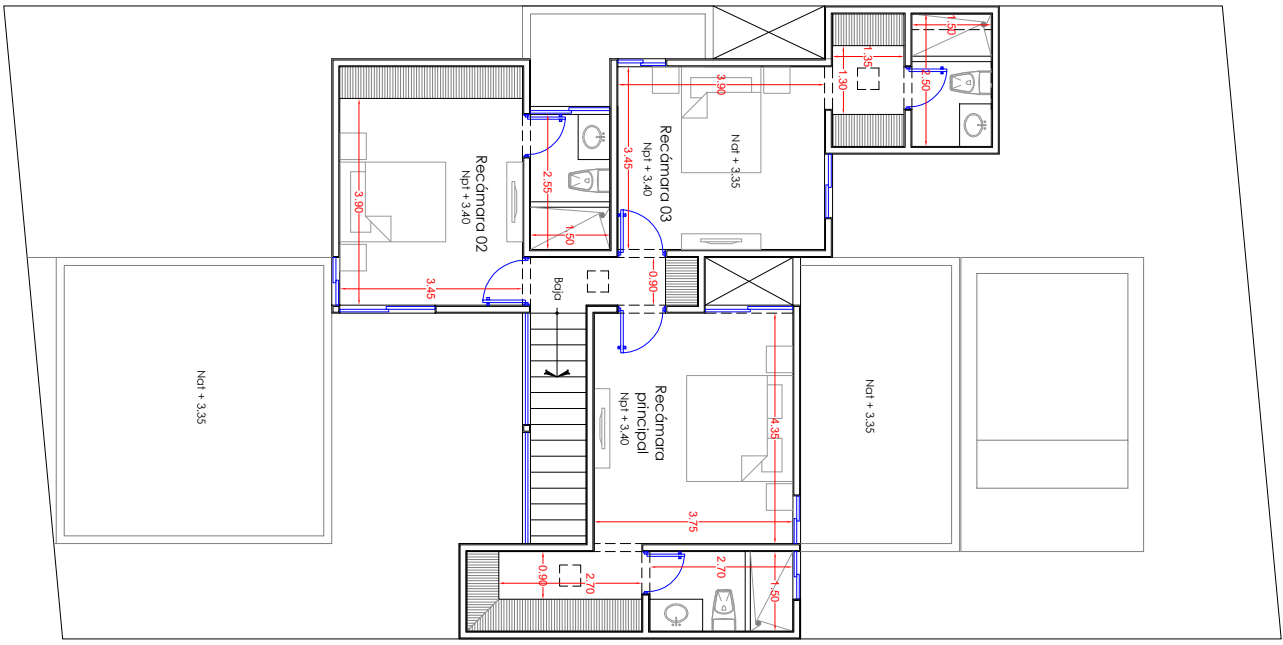
PLANTA ALTA
