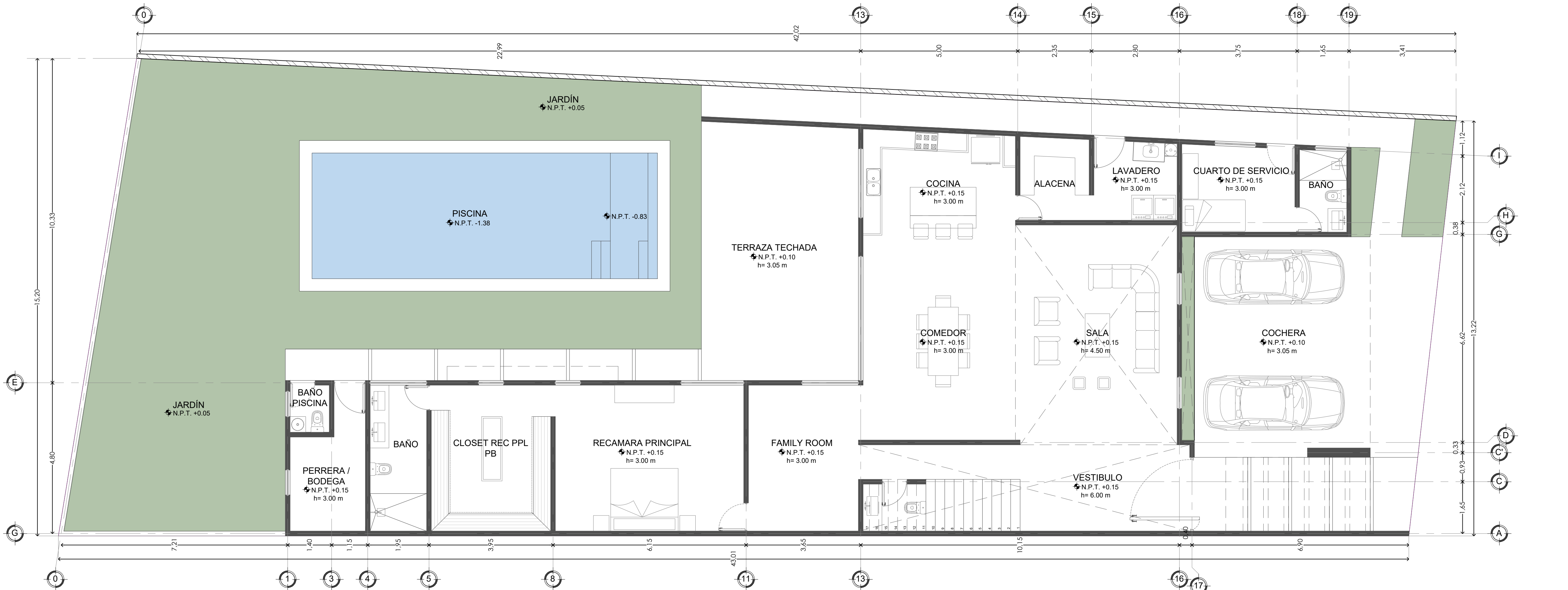
PLANTA BAJA Esc. 1:75 Acolación: Metros
